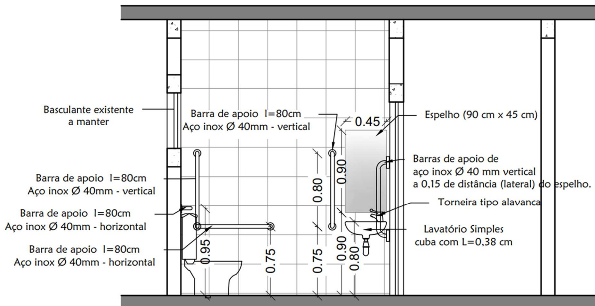
Figura 6 - Corte BB do banheiro Feminino com as medidas a serem utilizadas.
