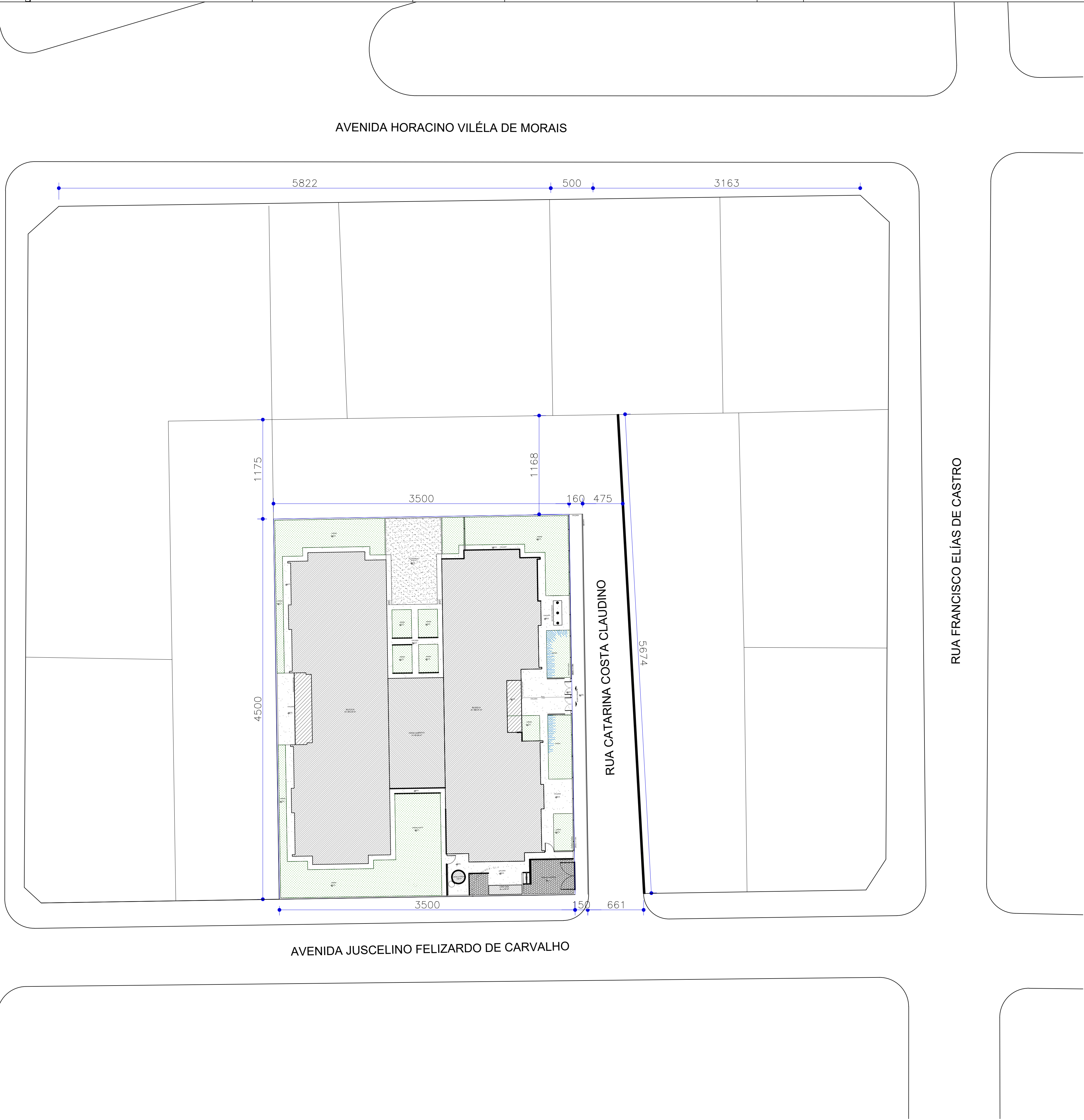
1 PLANTA DE IMPLANTAÇÃO ESCALA 1/250
