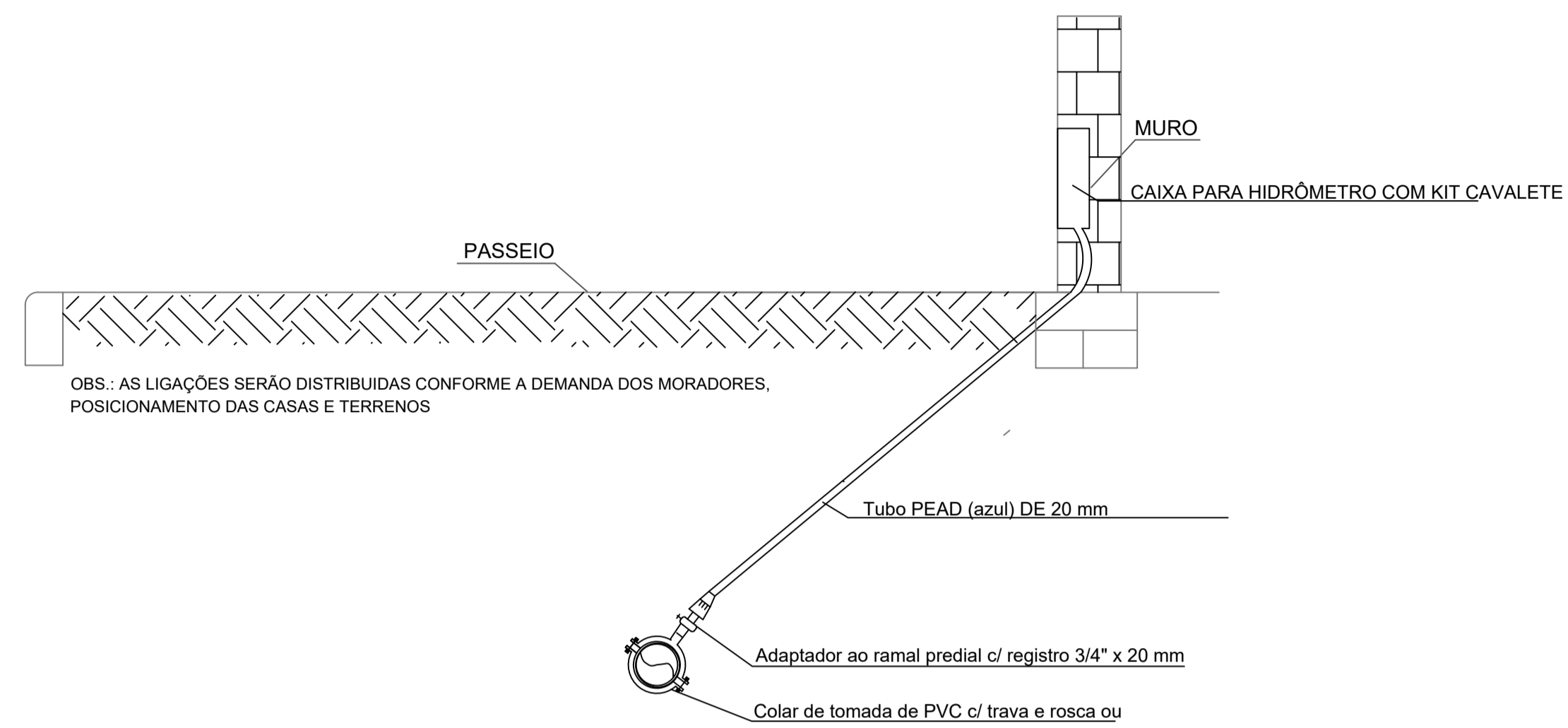
DETALHE LIGAÇÃO PREDIAL DE ÁGUA SEM ESCALA
