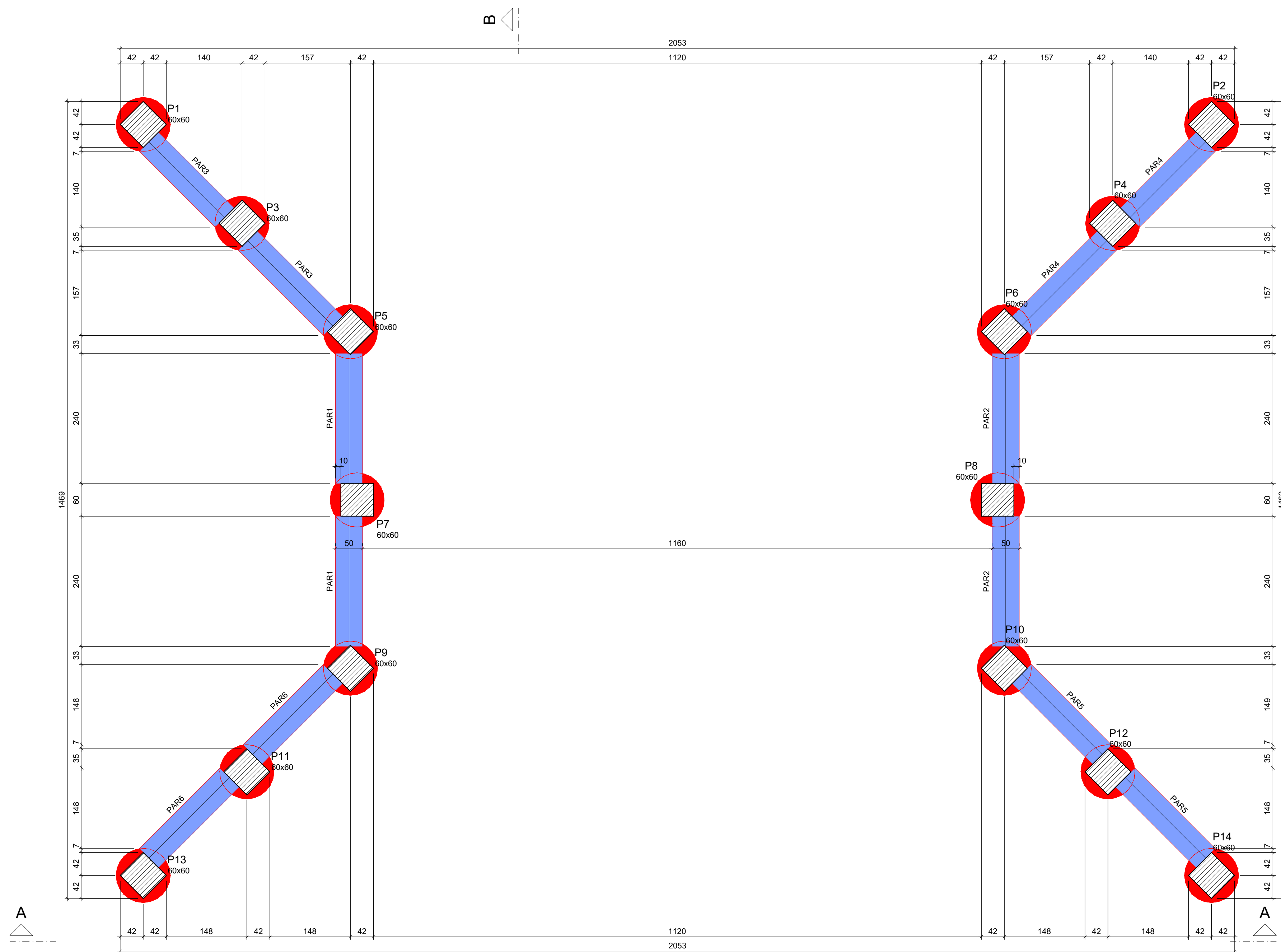
FORMA DO PAVIMENTO FUNDAÇÃO Escala 1:50
