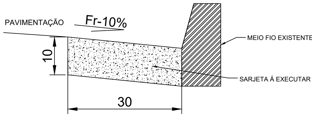
SEÇÃO DA SARJETA MEDIDAS EM CENTÍMETRO NOS BORDOS DA PAVIMENTAÇÃO PARA ESCOAMENTO DE ÁGUAS PLUVIAIS SERÁ CONSTRUÍDO SARJETA.
