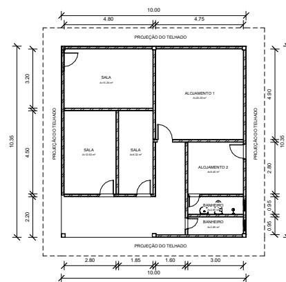
2 Levantamento 1 : 100
