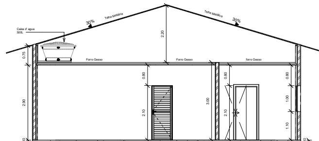
7 Corte BB 1 : 50
