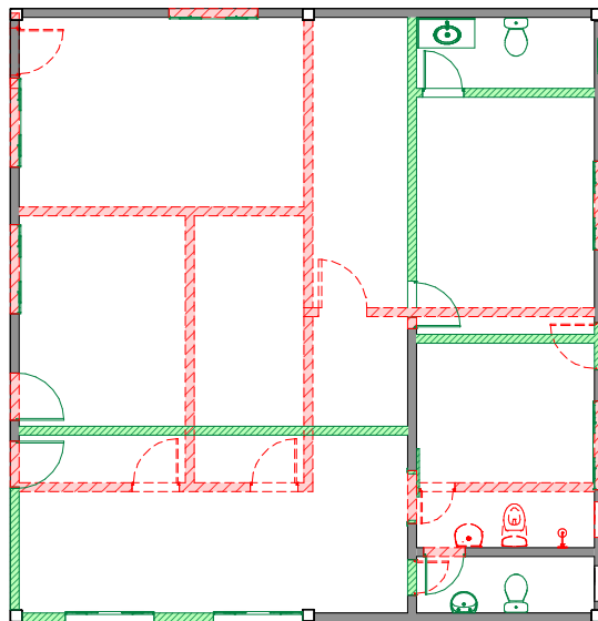
1 Planta Baixa Reforma 1 : 50
