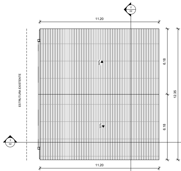
1 Cobertura 1 : 75
