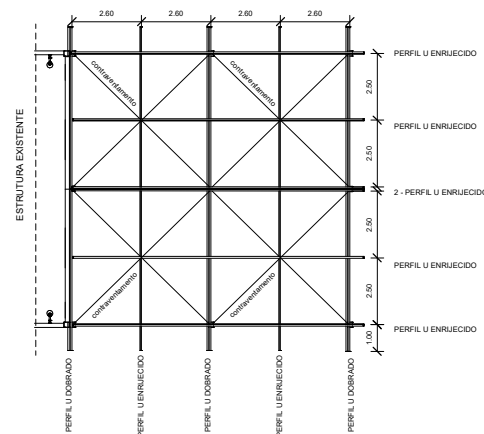
5 Estrutura do telhado 1 : 100
