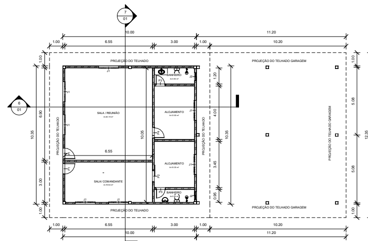
3 Projeto Final 1 : 100
