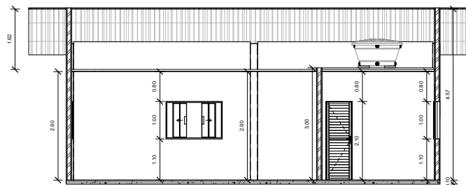
6 Corte AA 1 : 50
