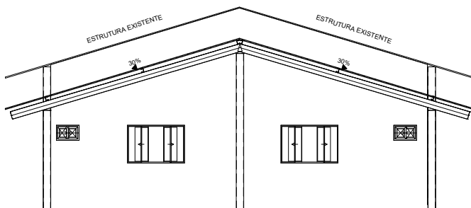
2 Corte A - Garagem 1 : 50
