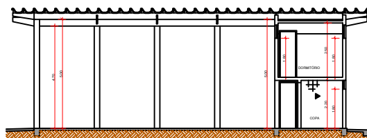
CORTE AA escala: 1/75
