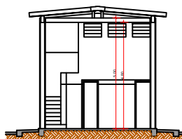
CORTE CC escala: 1/75
