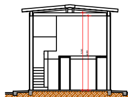
CORTE BB escala: 1/75
