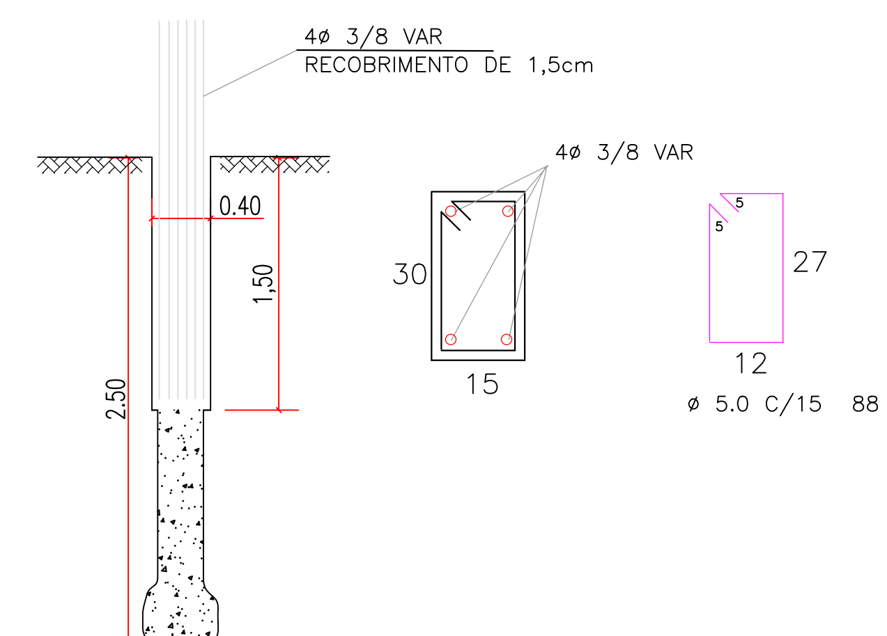
DET. DAS ESTACAS/PILARES
