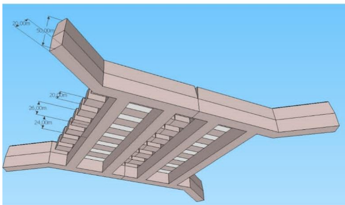
Imagem 01: Dimensões do mata-burro
