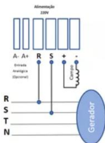
Ligação em 220V
