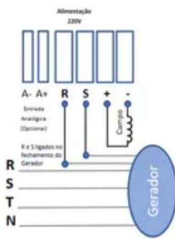
Ligação em 440V (ou 380V)
