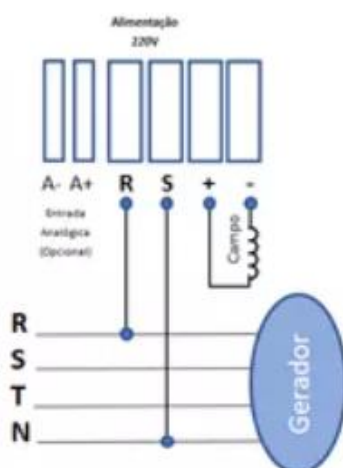
Ligação em 380V
