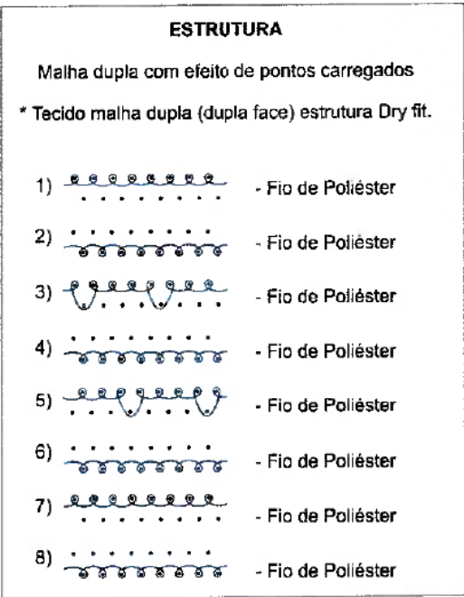
Figura 02 - Desenho técnico da estrutura da malha camuflada.
