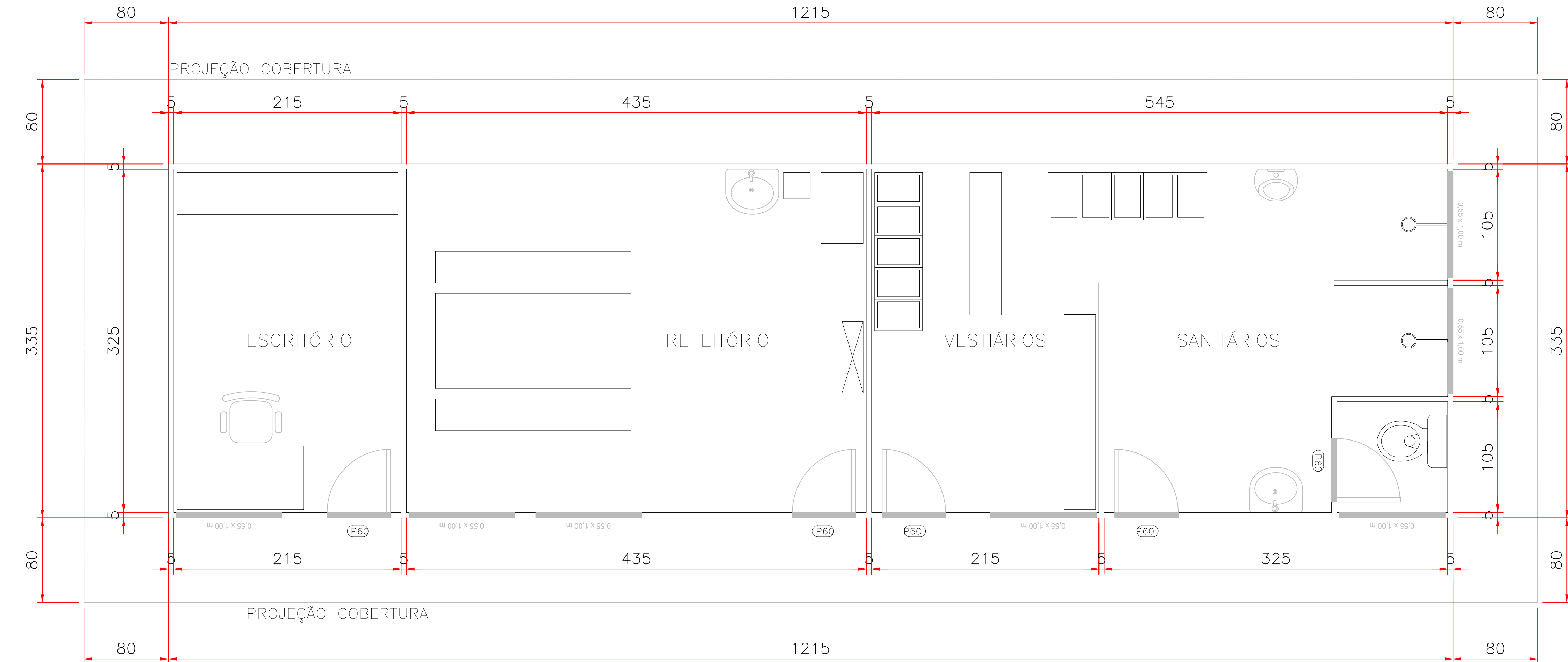
PLANTA LAYOUT DA ÁREA DE VIVENCIA DO CANTEIRO DE OBRA - TIPO II ESC 1:25
