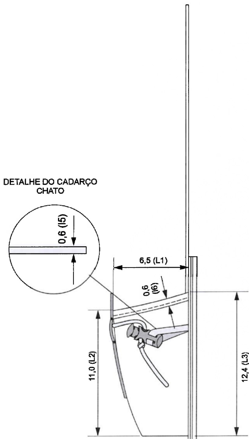
Figura 3 – Detalhes da lateral do Porta Carregador 7.62 mm / 5.56 mm
