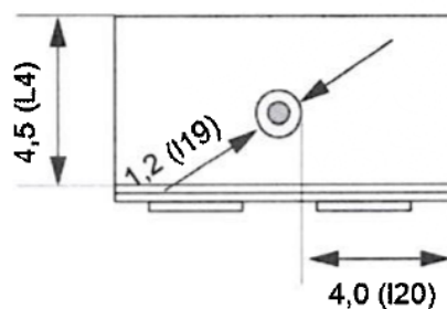
Figura 6 – Detalhes do fundo
