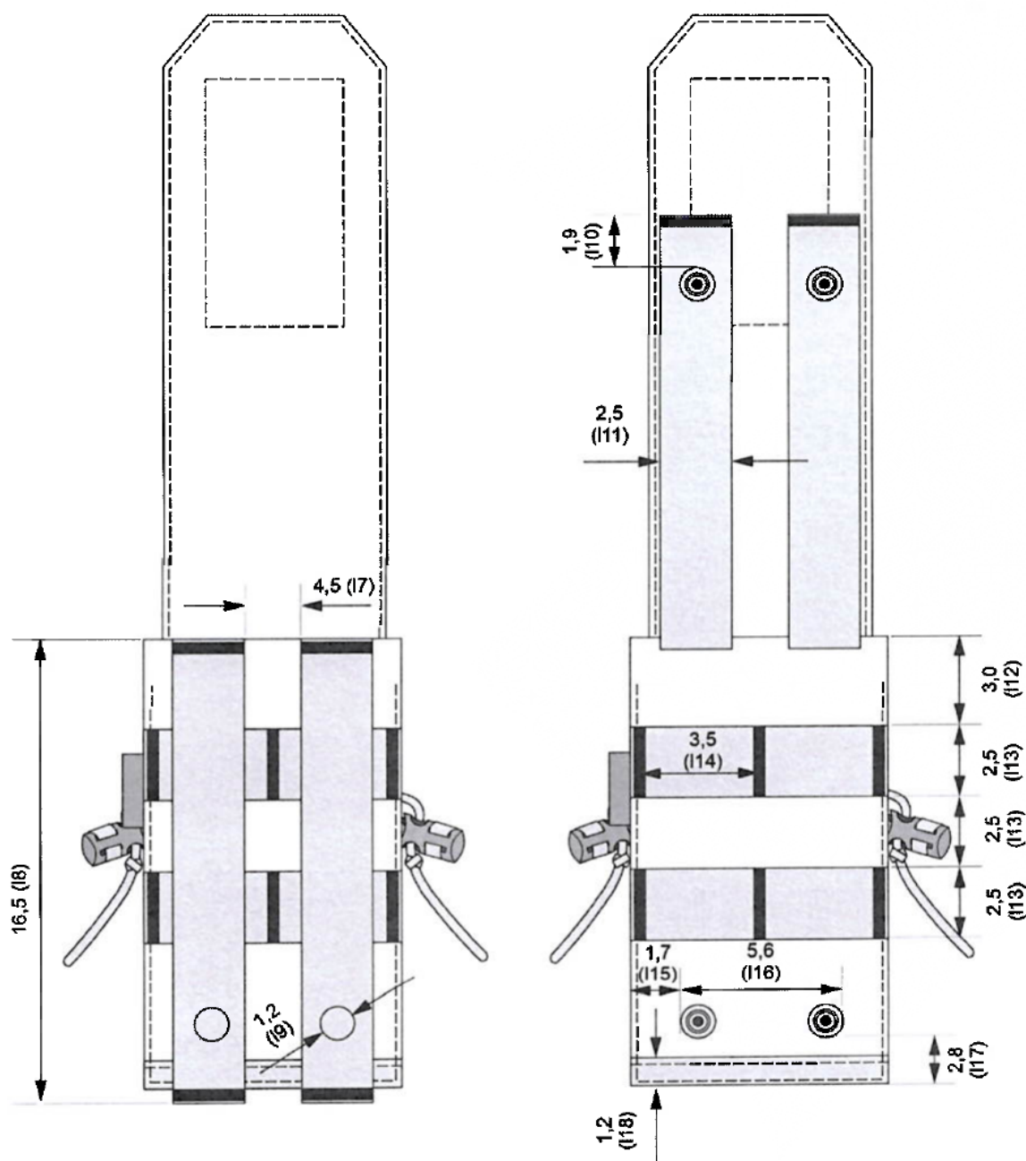
Figura 5 – Detalhes das costas com as alças levantadas
