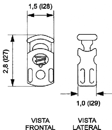
Figura 8 – Detalhes do regulador stopper do porta carregador 7.62 mm / 5.56 mm
