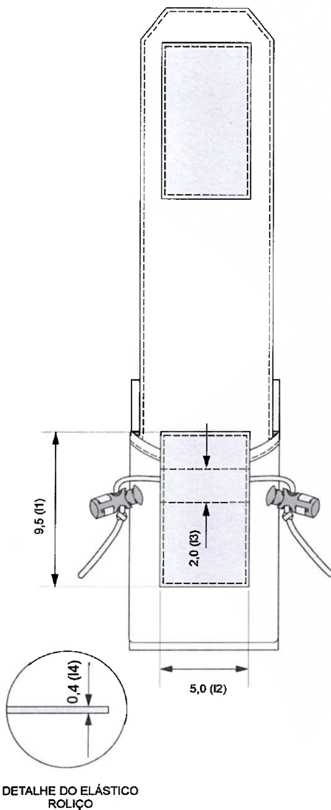
Figura 2 – Detalhes da frente do Porta Carregador 7.62 mm / 5.56 mm
