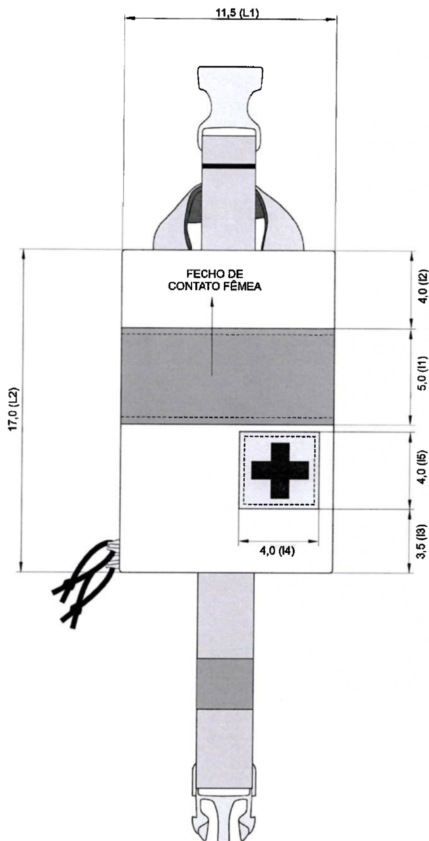
Figura 2 – Detalhes da frente do Porta KPSI Medidas em cm
