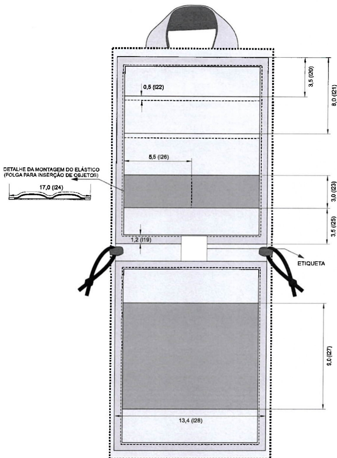
Figura 6– Detalhes da parte interna do Porta KPSI
