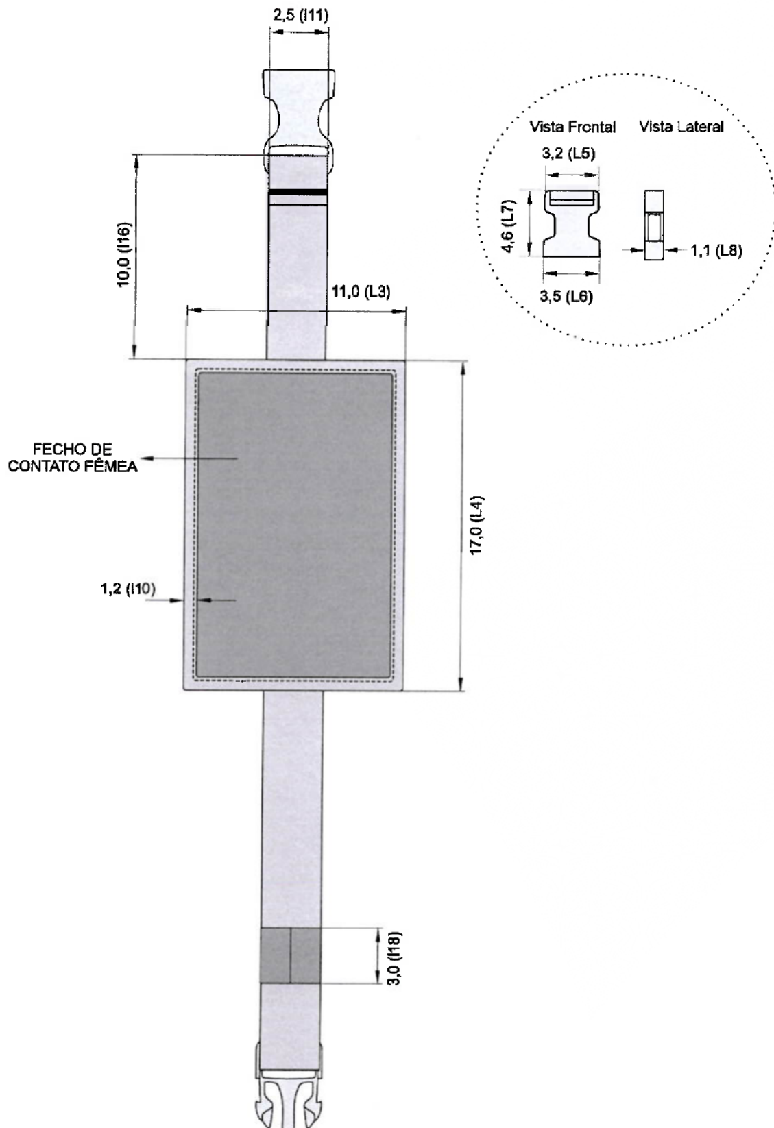
Figura 4 – Detalhes do lado interno da base de aplicação do Porta KPSI
