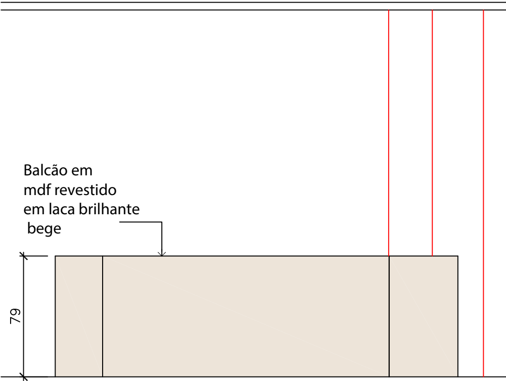
2 Balcão recepção – vista frontal 1/25
