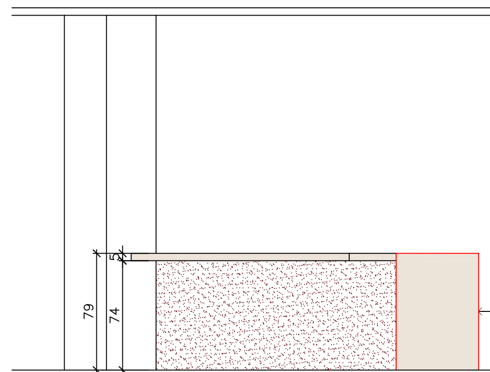
⑤ Balcão recepção – vista lateral 03 1/25
