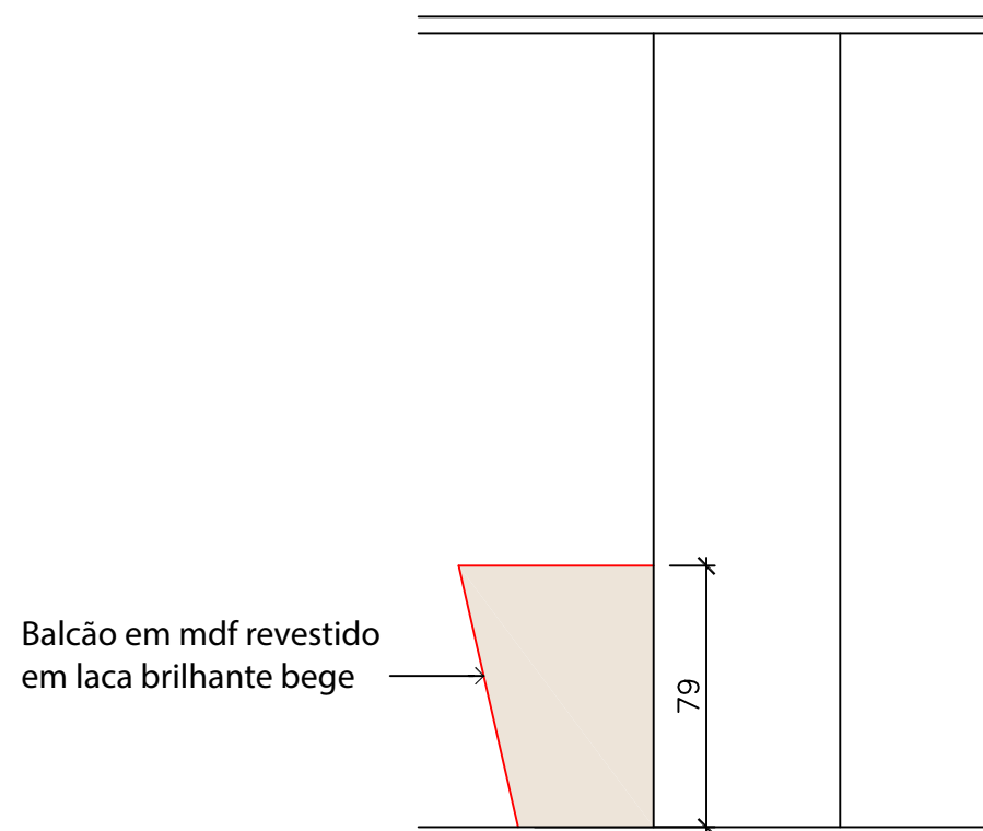
④ Balcão recepção – vista lateral 03 1/25
