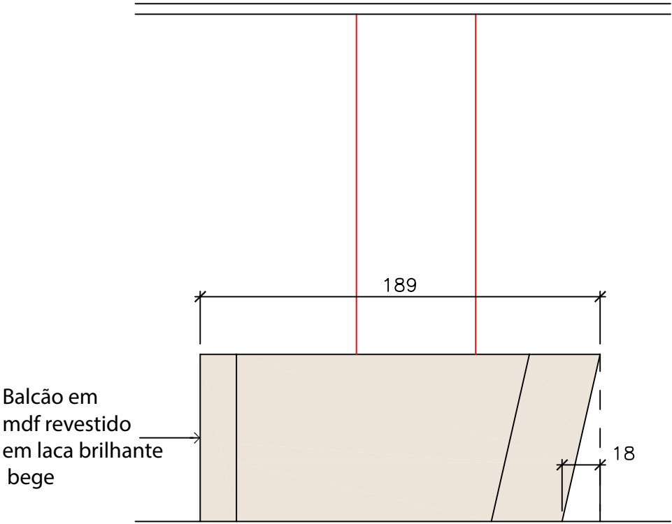
3 Balcão recepção – vista lateral 02 1/25
