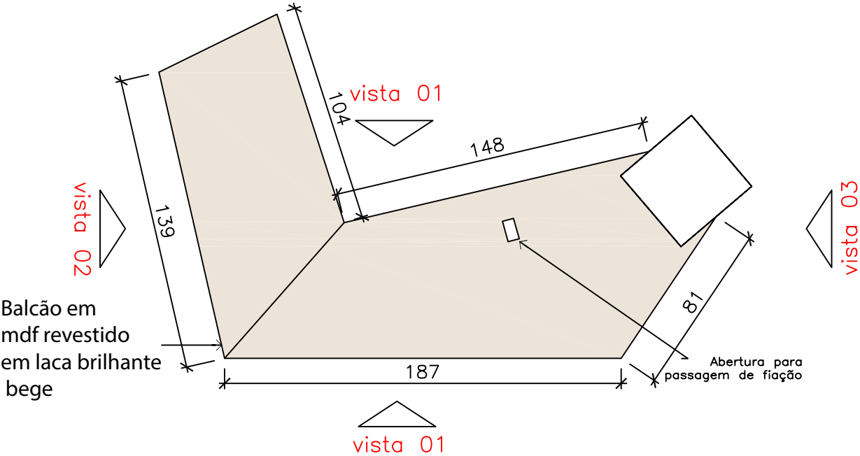
1 Balcão recepção – planta baixa 1/25
