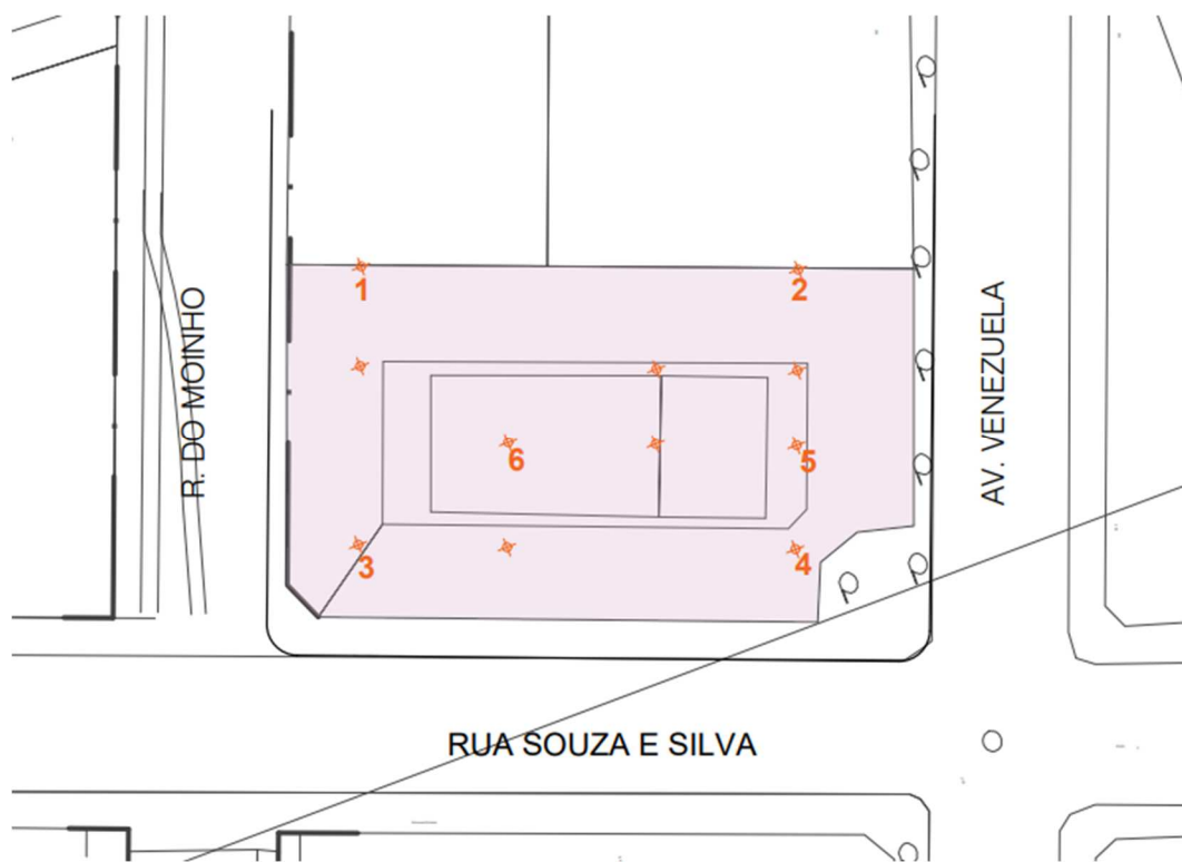
Figura 2- pontos de perfuração da sondagem SPT
