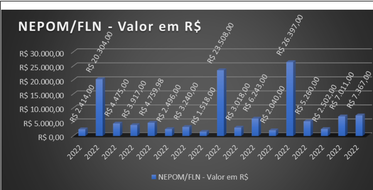
Gráfico 14 – Valores individualizados por ordem de serviço, gastos com manutenção das embarcações da flotilha do NEPOM de Florianópolis no ano de 2022.
