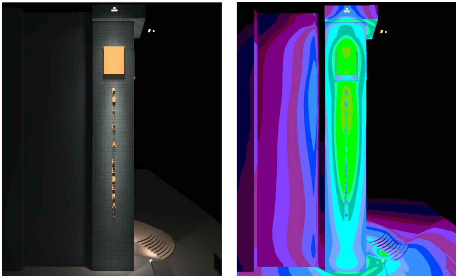
Fachada Lateral Representação da Iluminância e Gráfico das cores falsas. Fonte: Gerado pelas autoras no Software DIALux.
