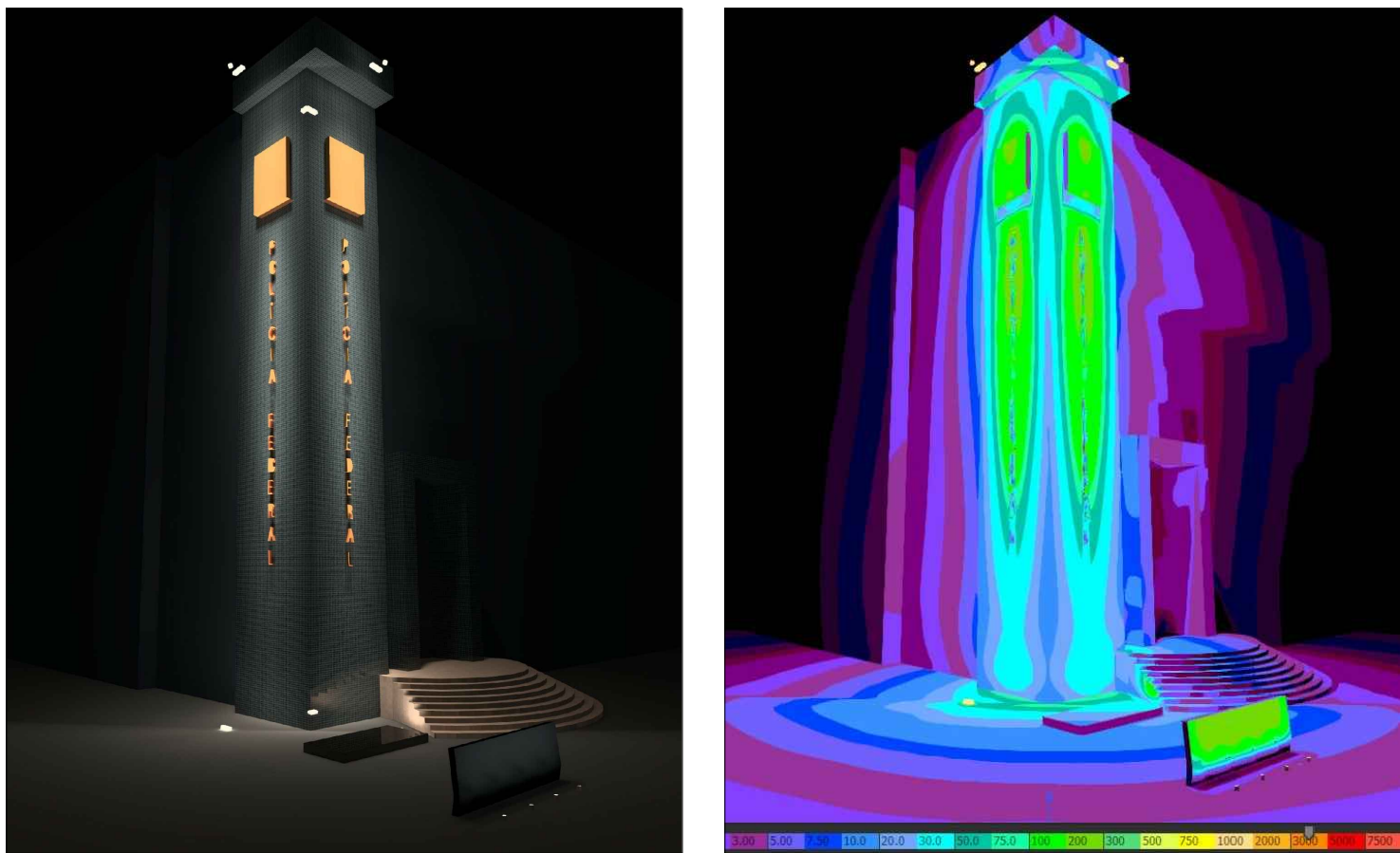
Fachada Frontal e Lateral Representação da Iluminância e Gráfico das cores falsas. Fonte: Gerado pelas autoras no Software DIALux.
