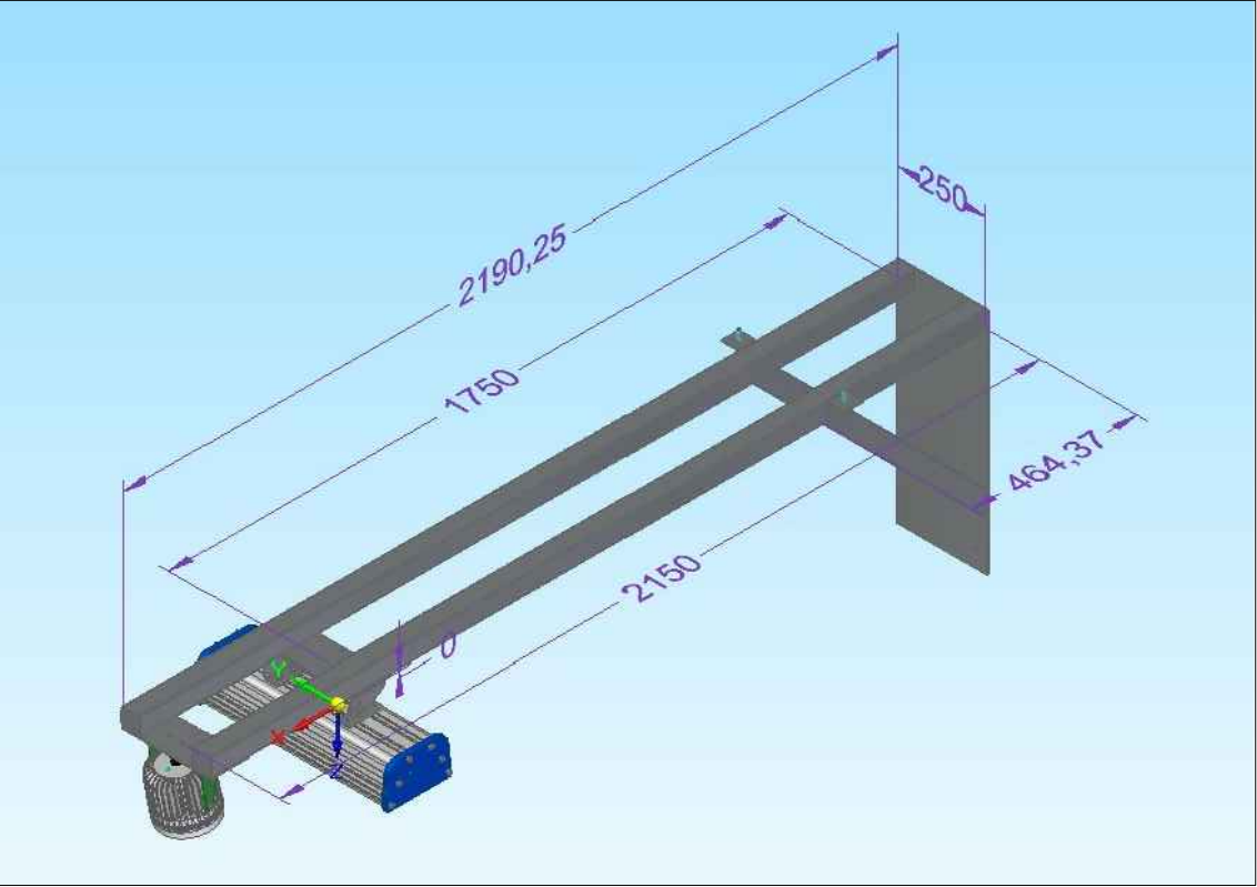
Suporte paraos projetores aéreos . Fonte: Powerlume.
