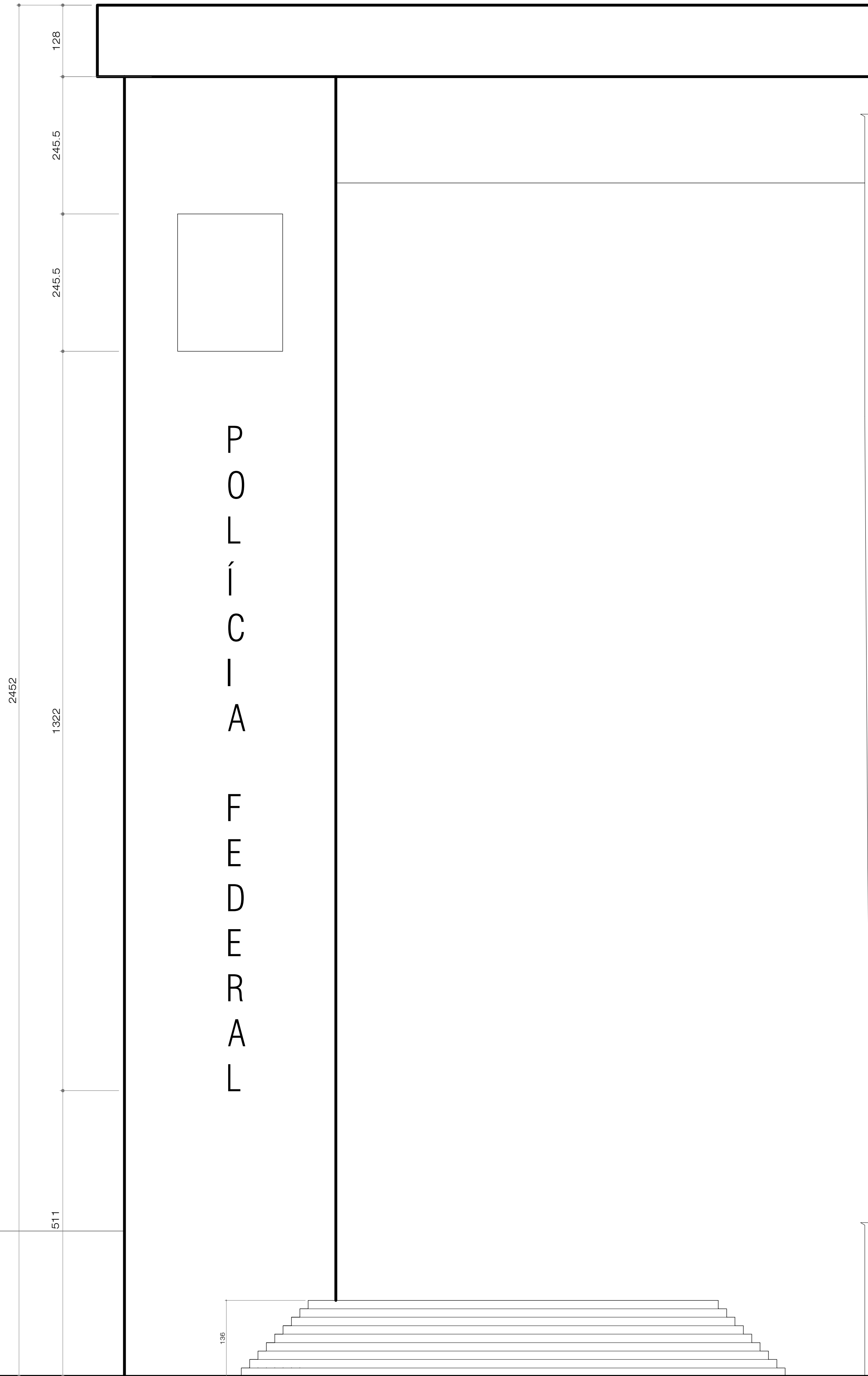
Vista 1 Levantamento Edificação Principal Escala 1:50
