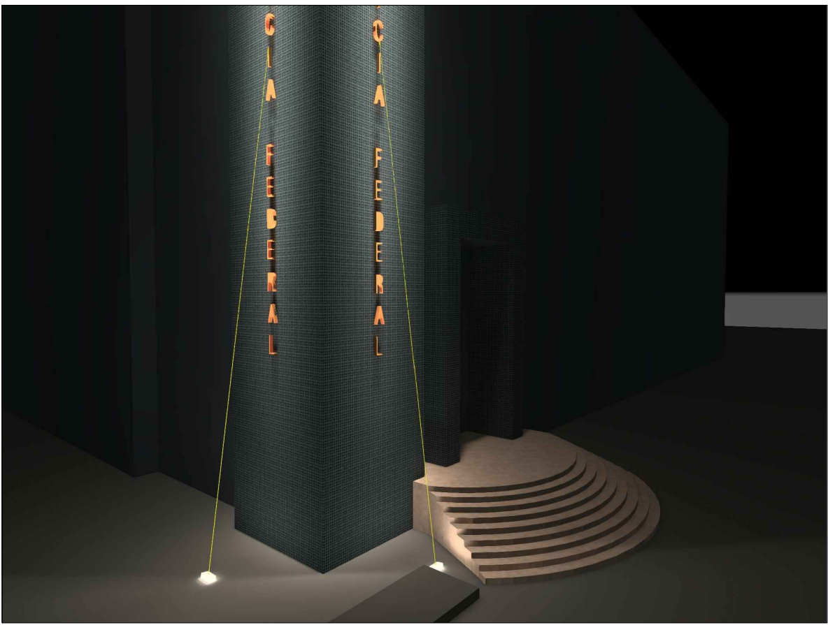
Fachadas Frotal e Lateral Direcionamento dos projetores no solo. Fonte: Gerado pelas autoras no Software DIALux.
