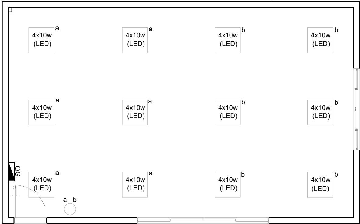
PLANTA BAIXA - INSTALAÇÕES ELÉTRICAS (ILU) ESCALA 1:50 A: 43,60m² A: 27,22m
