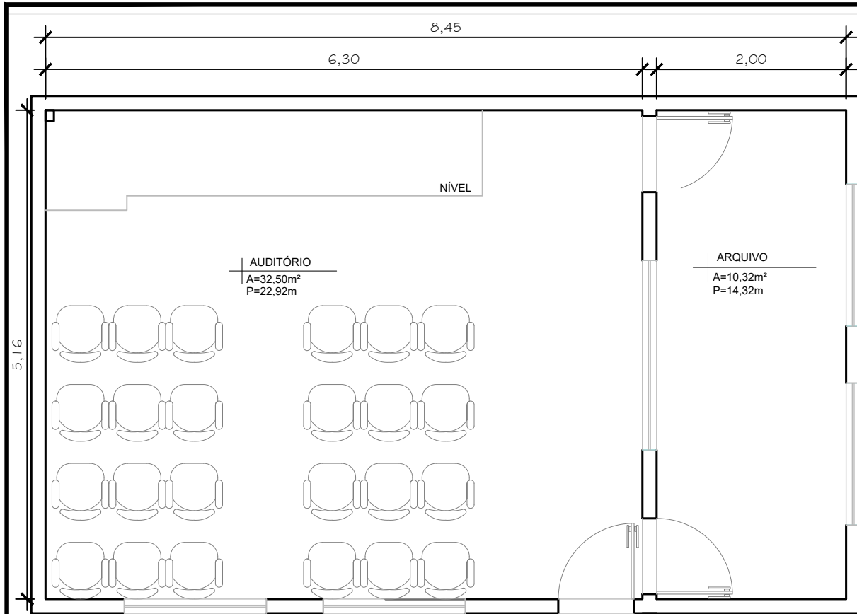
PLANTA-BAIXA EXISTENTE ESCALA 1:50 A: 43,60m² P: 27,22m
