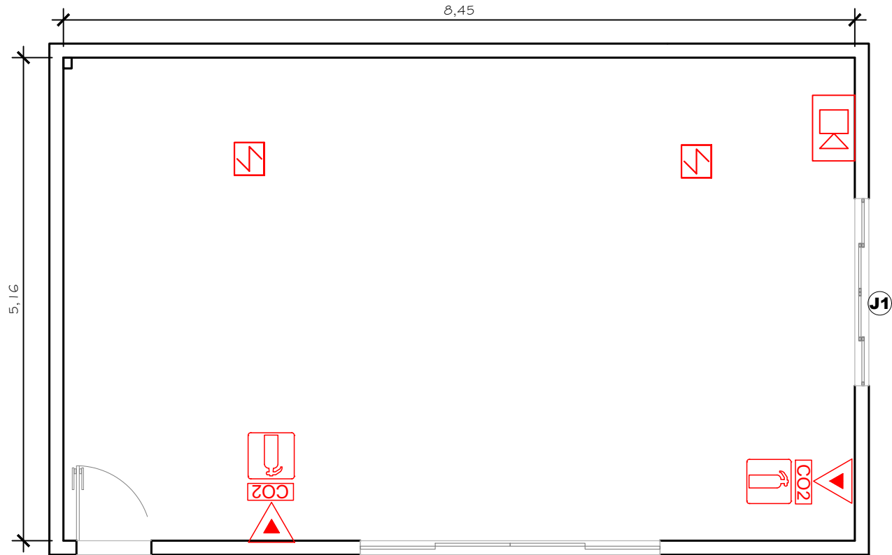
PLANTA BAIXA -COMBATE À INCÊNDIO ESCALA 1:50 A: 43,60m² A: 27,22m
