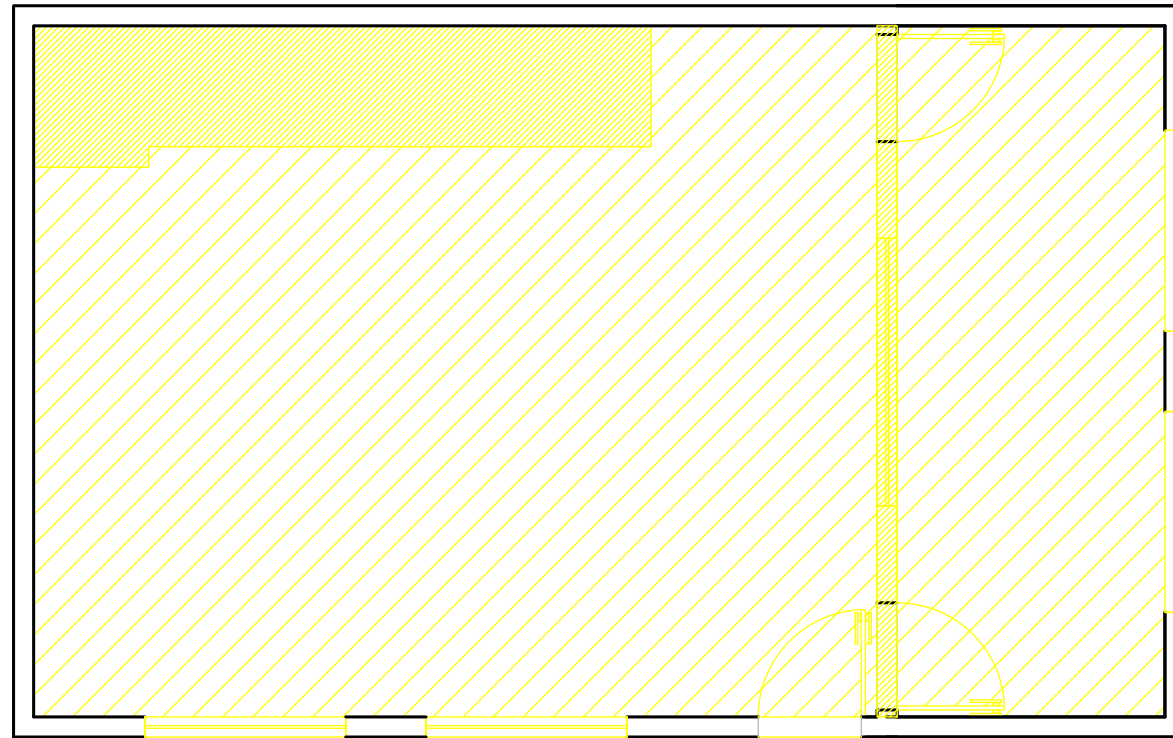
PLANTA BAIXA À DEMOLIR ESCALA 1:50 A: 43,60m² ■ À DEMOLIR (PISO, ESQUADRIA, FORRO) ■ À PERMANECER
