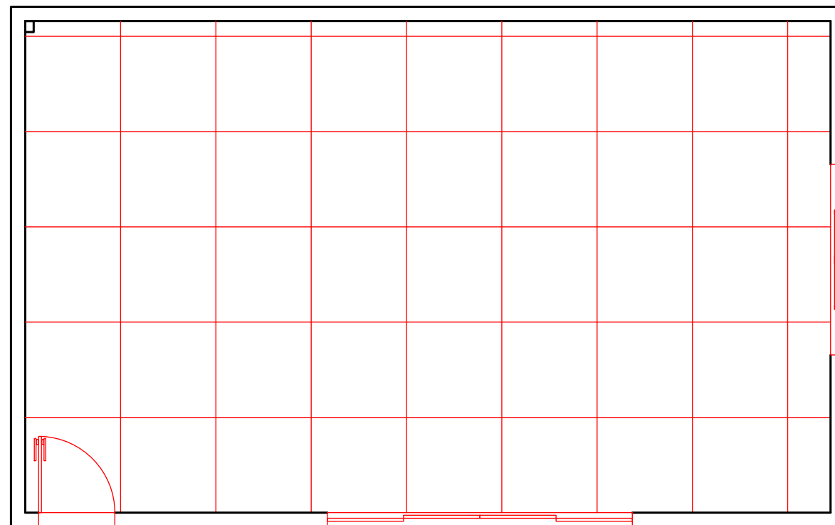
PLANTA-BAIXA À CONSTRUIR ESCALA 1:50 A: 43,60m² P: 27,22m ■ À CONSTRUIR (PISO, EQUADRIA, FORRO)
