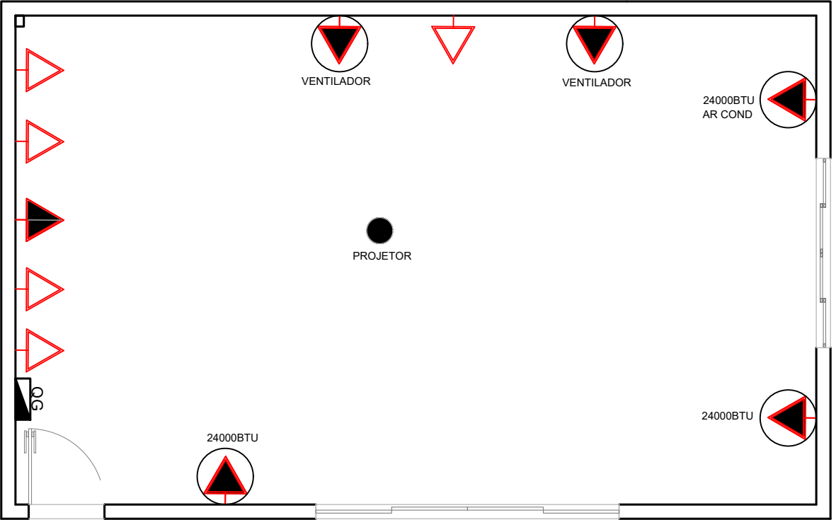
PLANTA BAIXA -INSTALAÇÕES ELÉTRICAS (TUG, TUE) ESCALA 1:50 A: 43,60m² A: 27,22m
