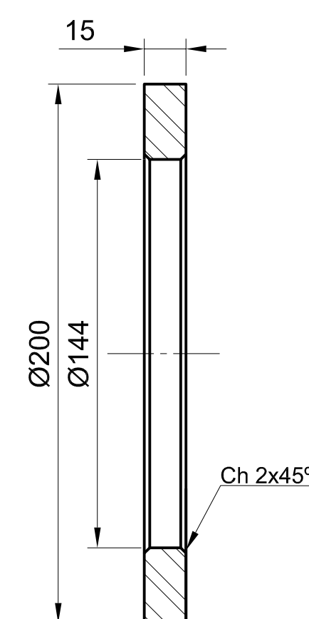
ANEL DE ESCORA (14) AÇO ASTM A-36 ESC: 1:2
