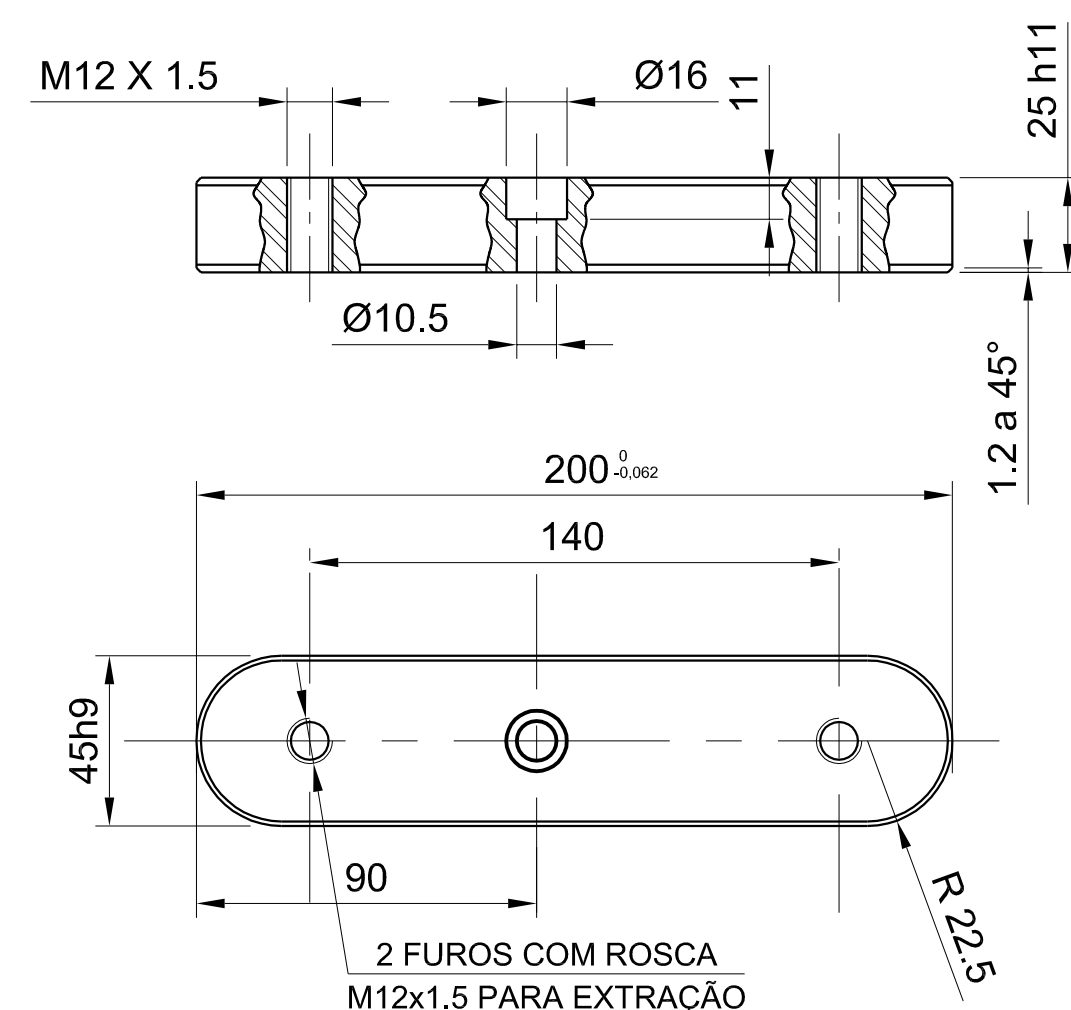
CHAVETA (27) AÇO CARBONO 1045 ESC: 1:2
