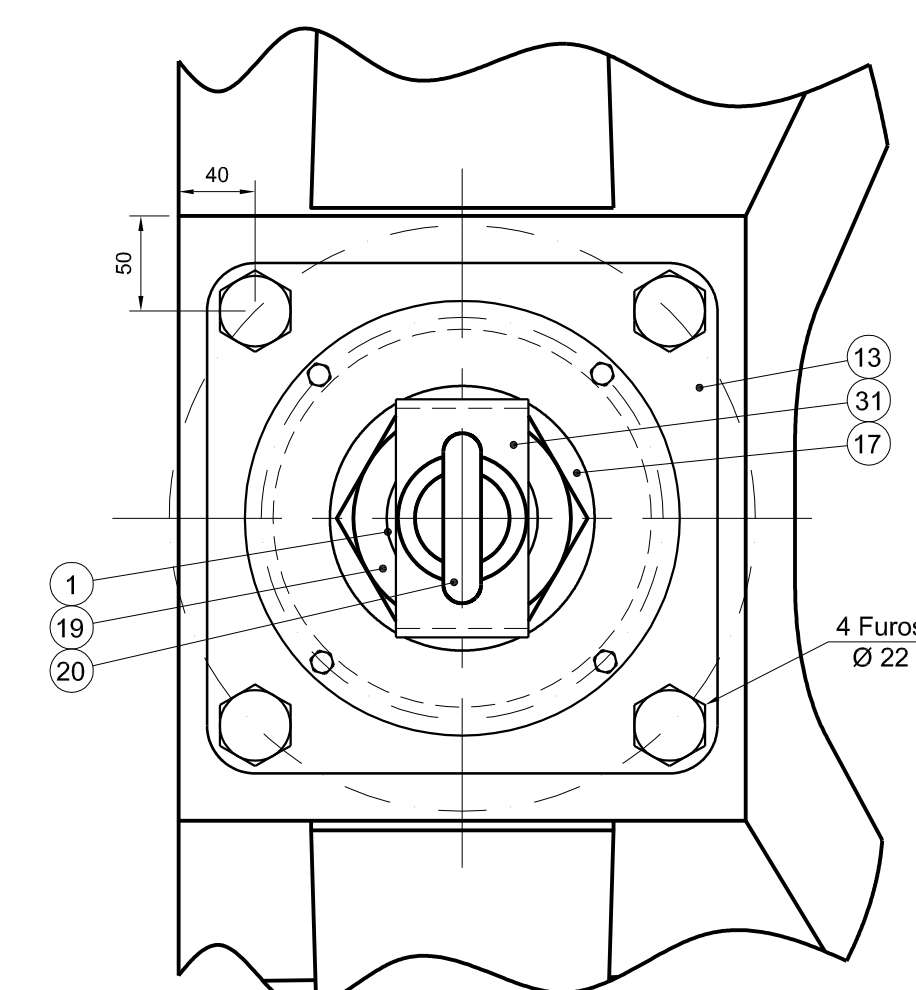
DETALHE DE MONTAGEM DA CAIXA DE ROLAMENTO NA ESTRUTURA (Sem Escala)
