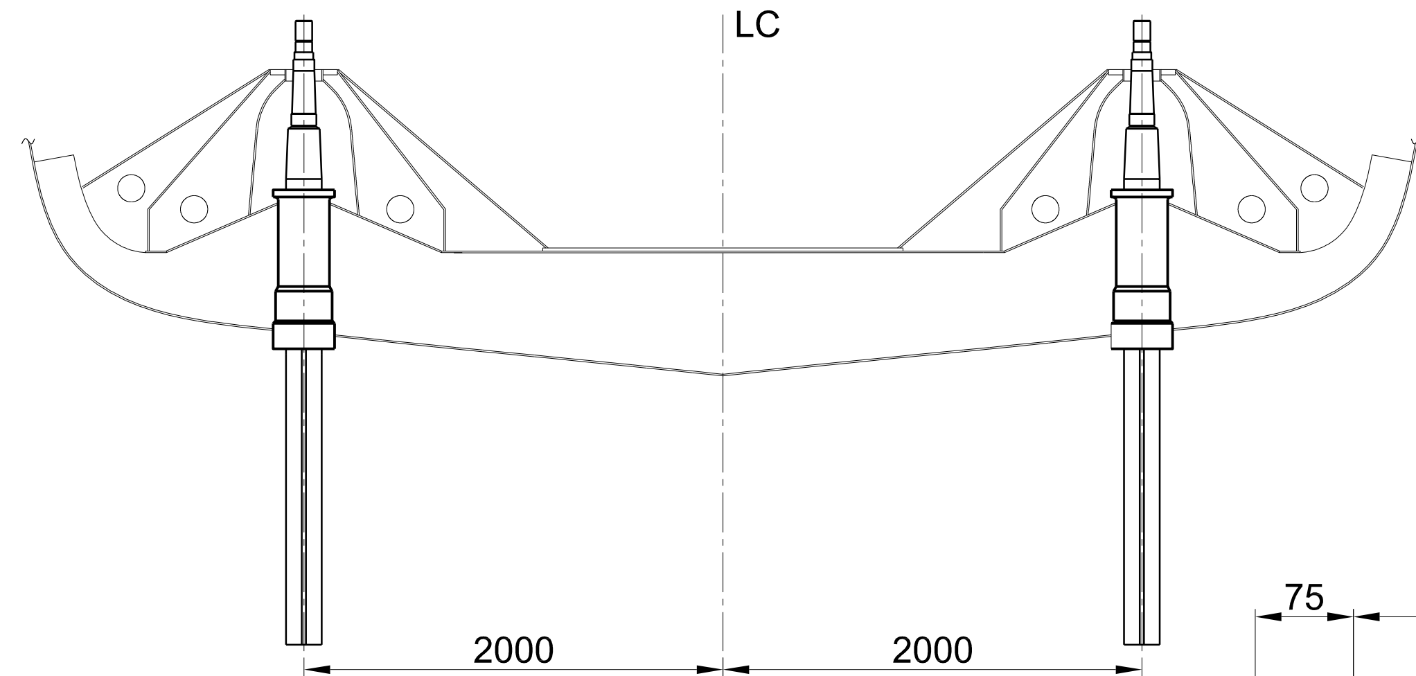
Vista na Cav. 1.8 olhando para vante Escala 1 / 25
