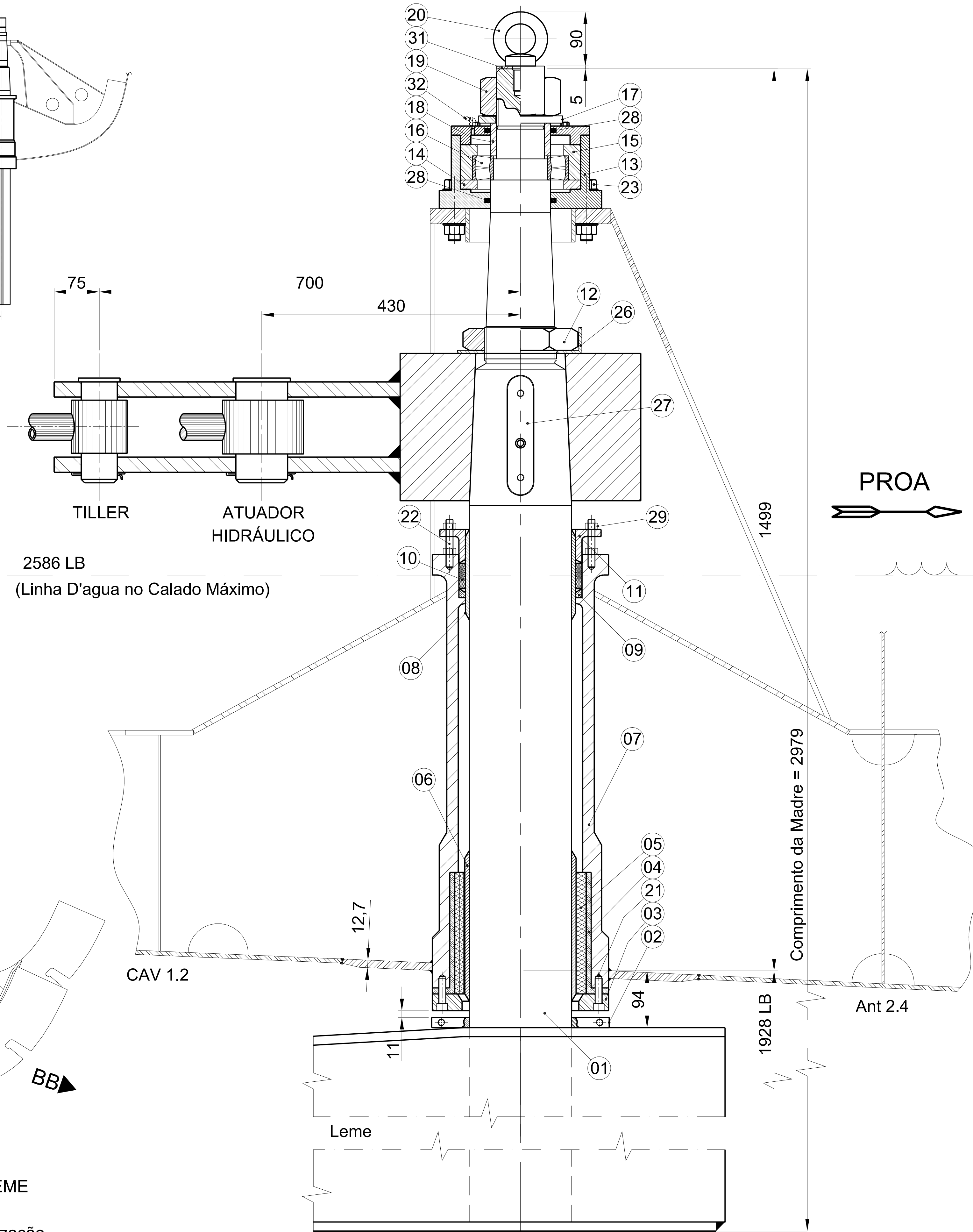
Corte Longitudinal a 2000 LC Escala 1 / 4
