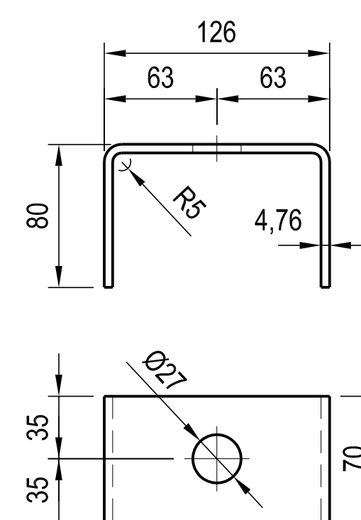
TRAVA DA PORCA DA MADRE (31) ESC: ____ 1:3
