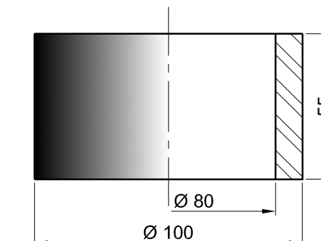
ANEL INTERNO (18) ESC: ____ 1:2
