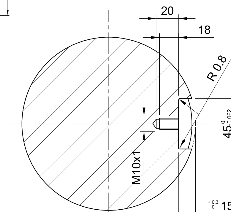
CORTE B-B' ESC: 1:2
