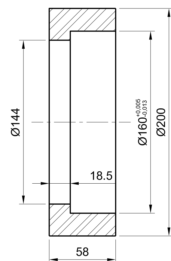
BUCHA INTERNA (15) AÇO ASTM A-36 ESC: 1:2
