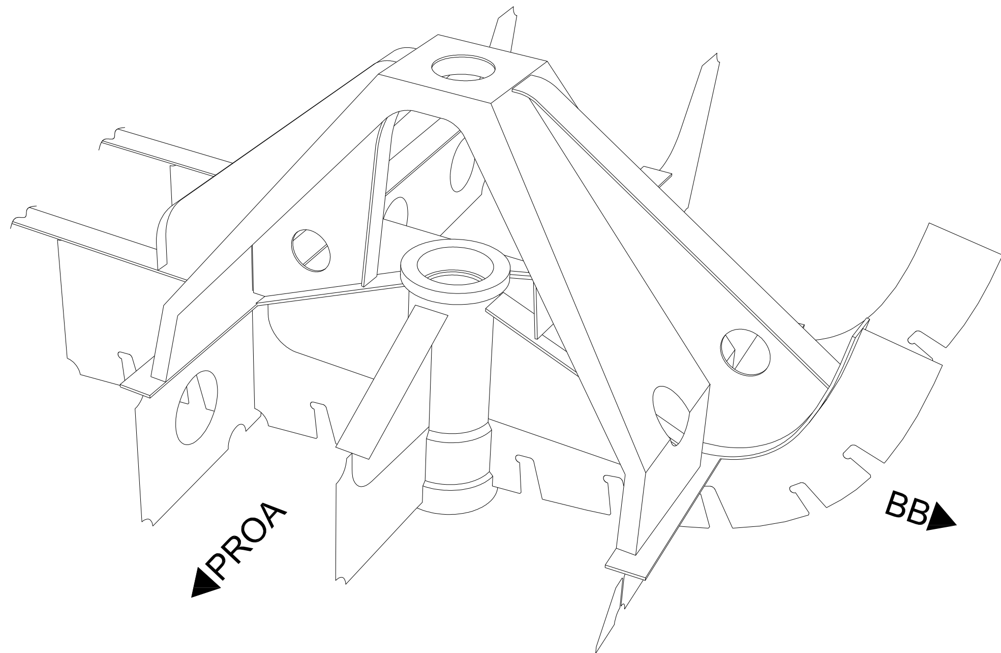
ESTRUTURA PARA MONTAGEM DA MÁQUINA DO LEME (Sem Escala) Nota: As partes móveis foram removidas para melhor vizualização.
