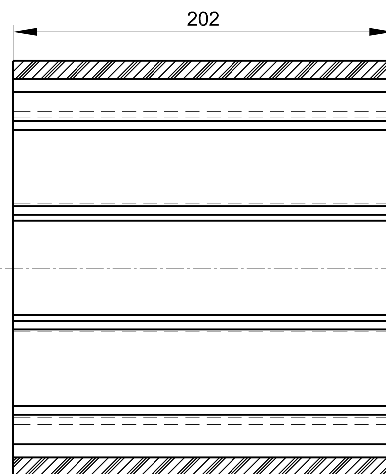
CORTE B-B'
