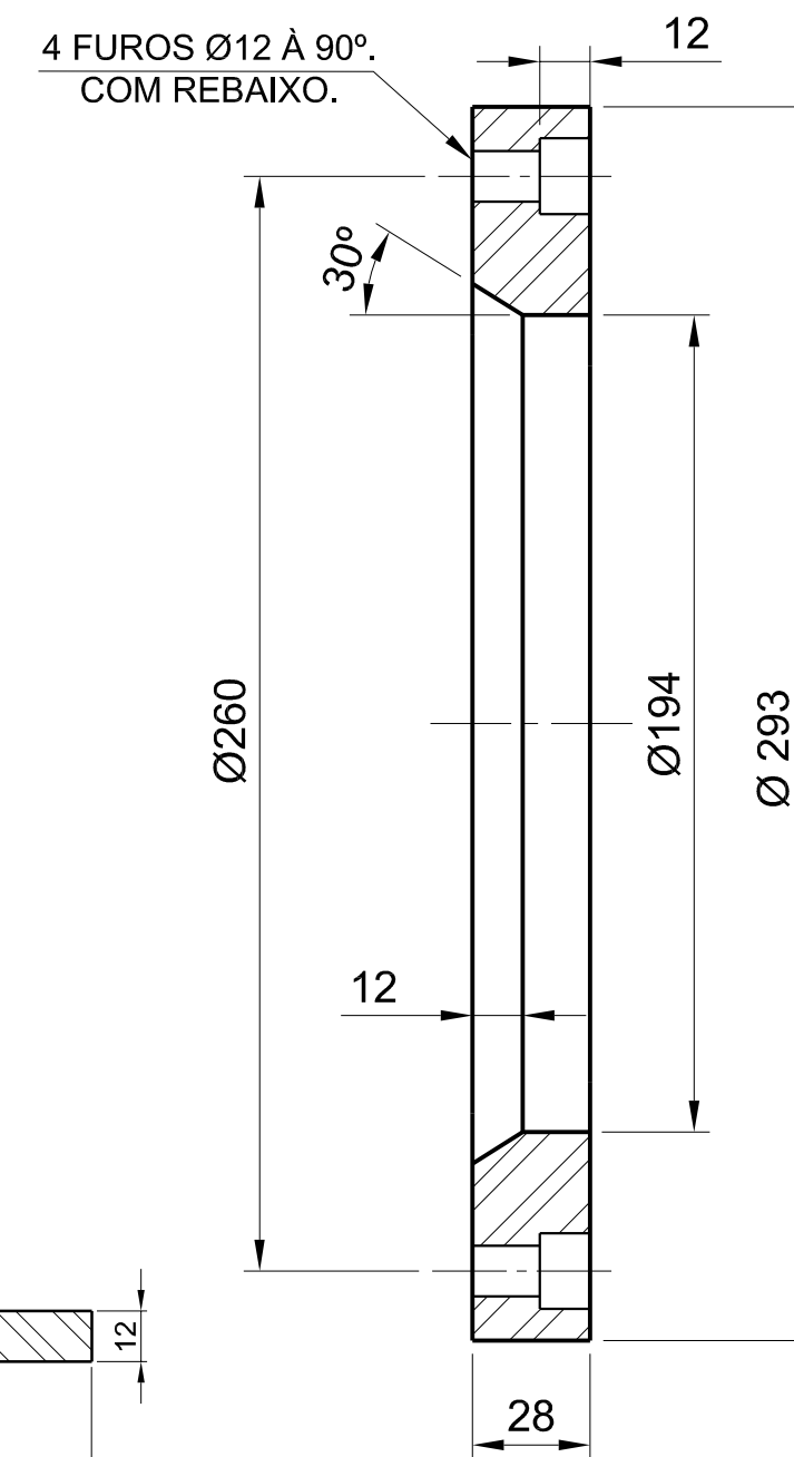
FLANGE DE FIXAÇÃO (03) AÇO ASTM A-36 ESC: 1:2
