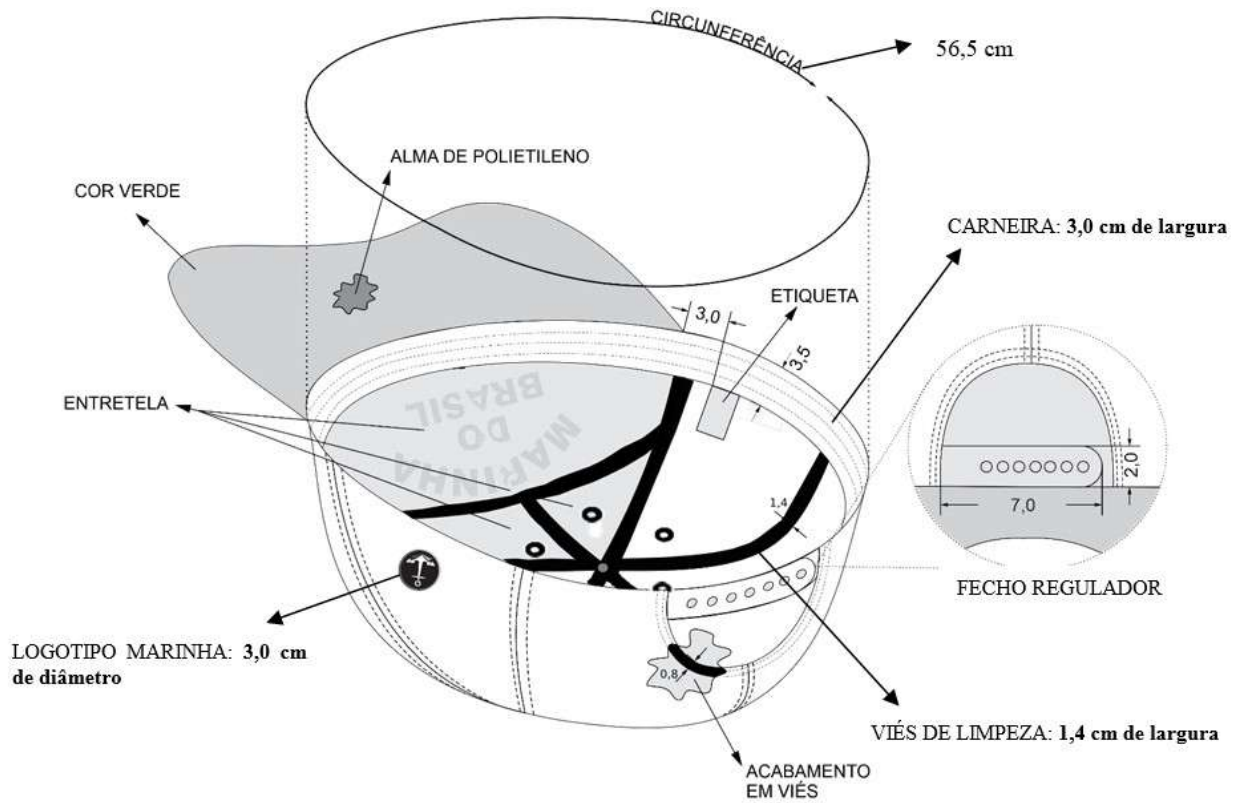
Figura 3 – Medidas do gorro em cm (parte interna e externa)
