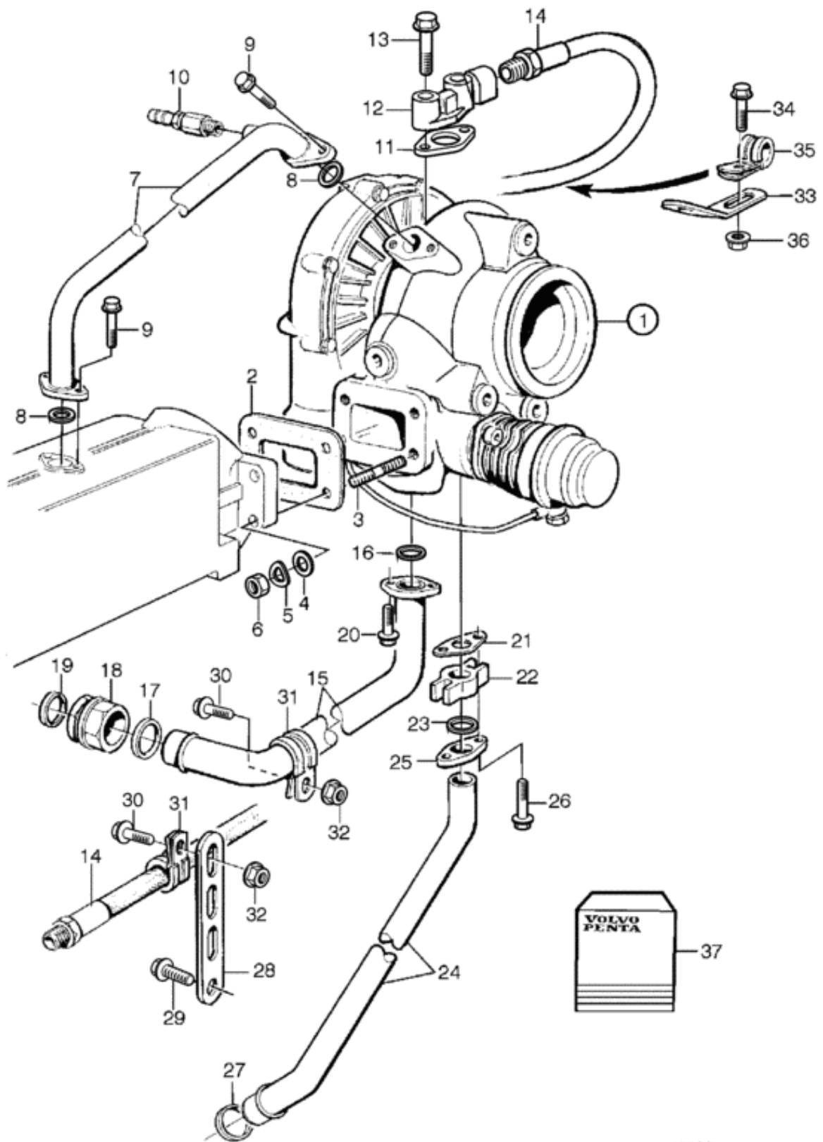
FIGURA 5 - ITEM 5 - GAXETA - PART NUMBER 831622 - PEÇA 08
