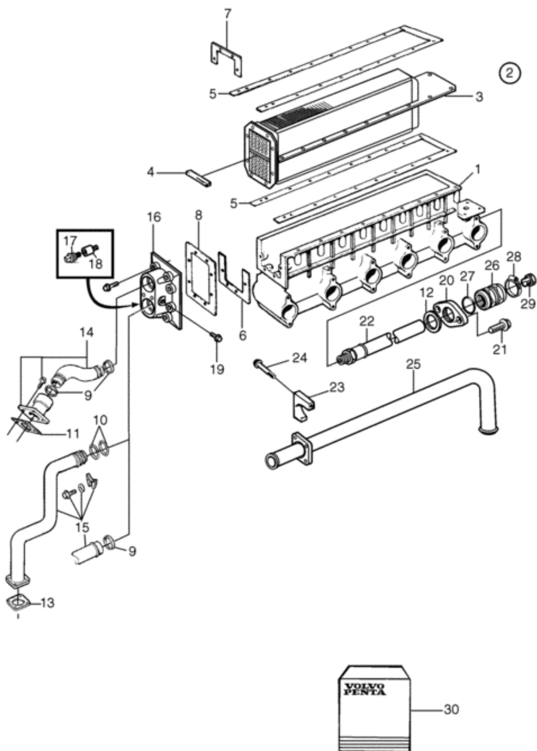
FIGURA 8 - ITEM 8 - ANODO MOTOR - PART NUMBER 838929 - PEÇA 18
