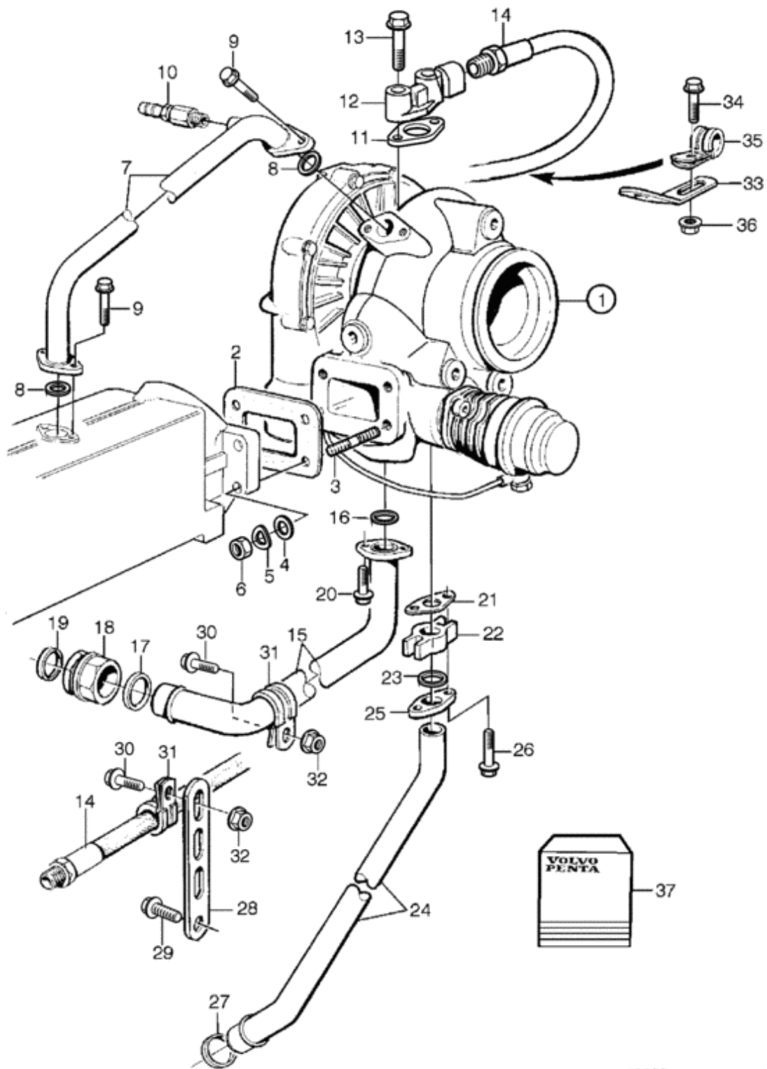
FIGURA 4 - ITEM 4 - ANEL DE BORRACHA - PART NUMBER 471626 - PEÇA 17
