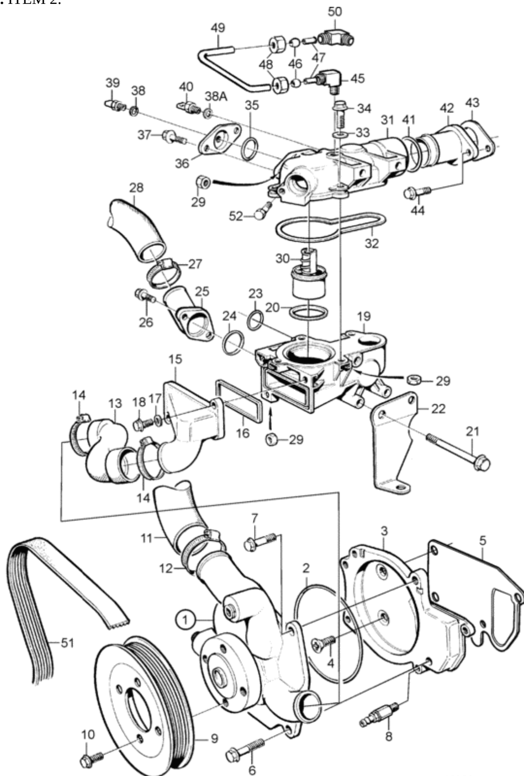
FIGURA 2 - ITEM 2 - MANGUEIRA - PART NUMBER 866216 - PEÇA 11
