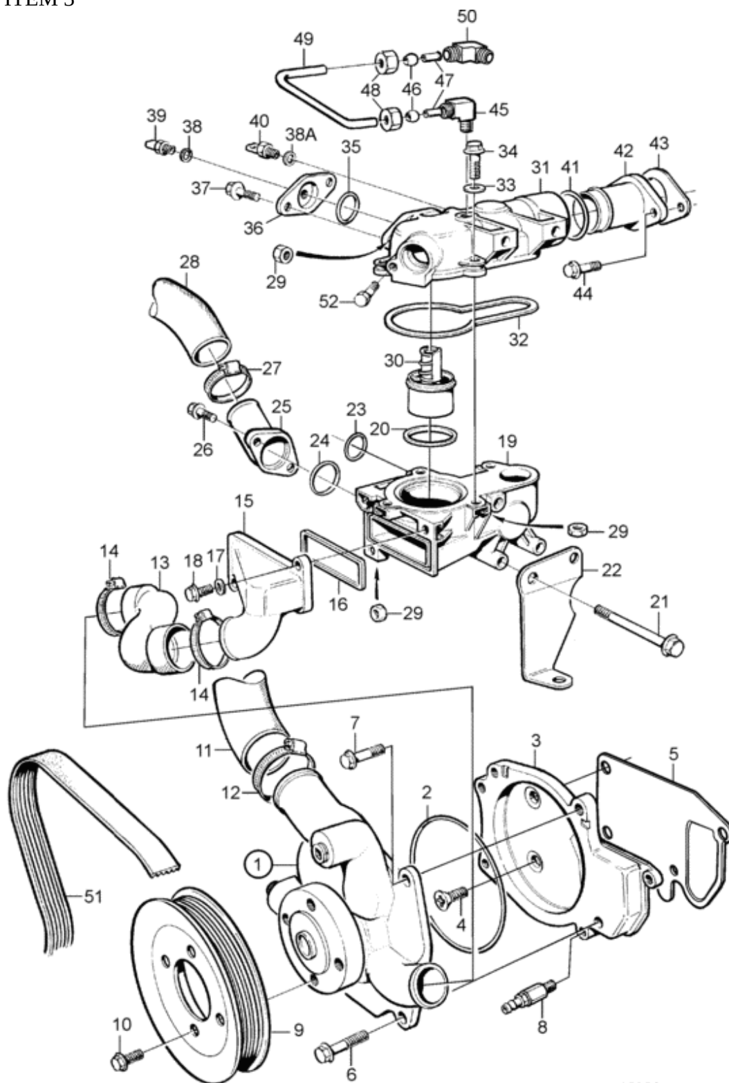
FIGURA 3 - ITEM 3 - MANGUEIRA - PART NUMBER 866215 - PEÇA 28
