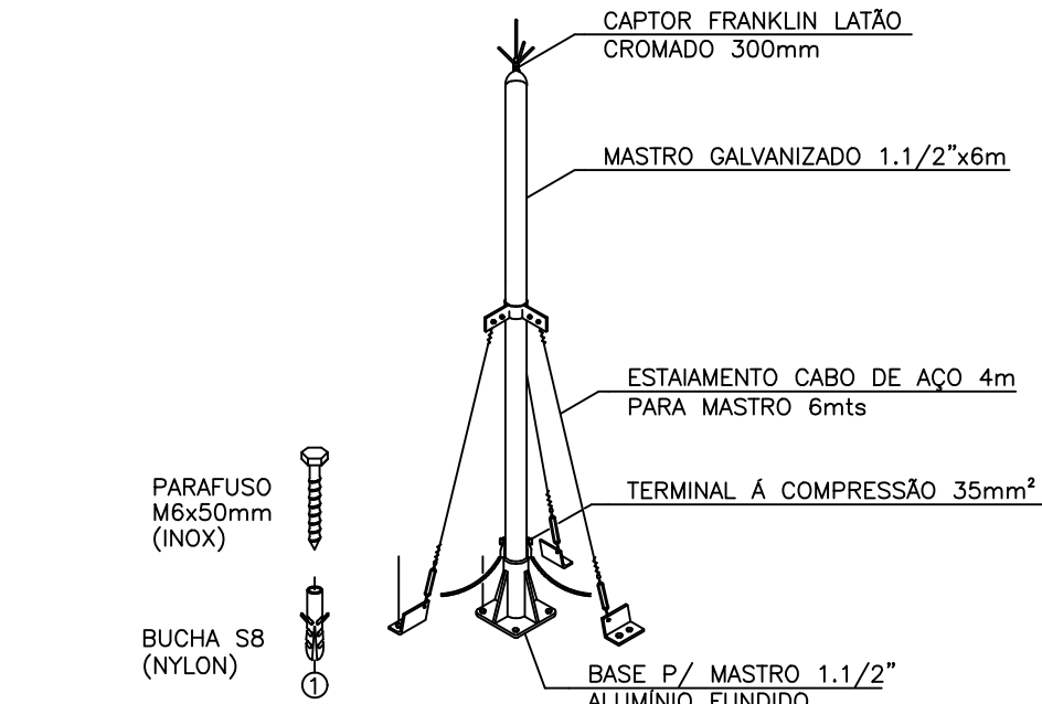
DETALHE DE INSTALAÇÃO MASTRO CAPTOR COM ESTAIAMENTO EM CABO DE AÇO H=6m
