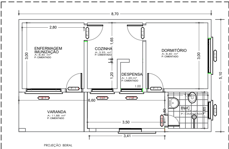
PLANTA BAIXA EXISTENTE - PARALELO 10
