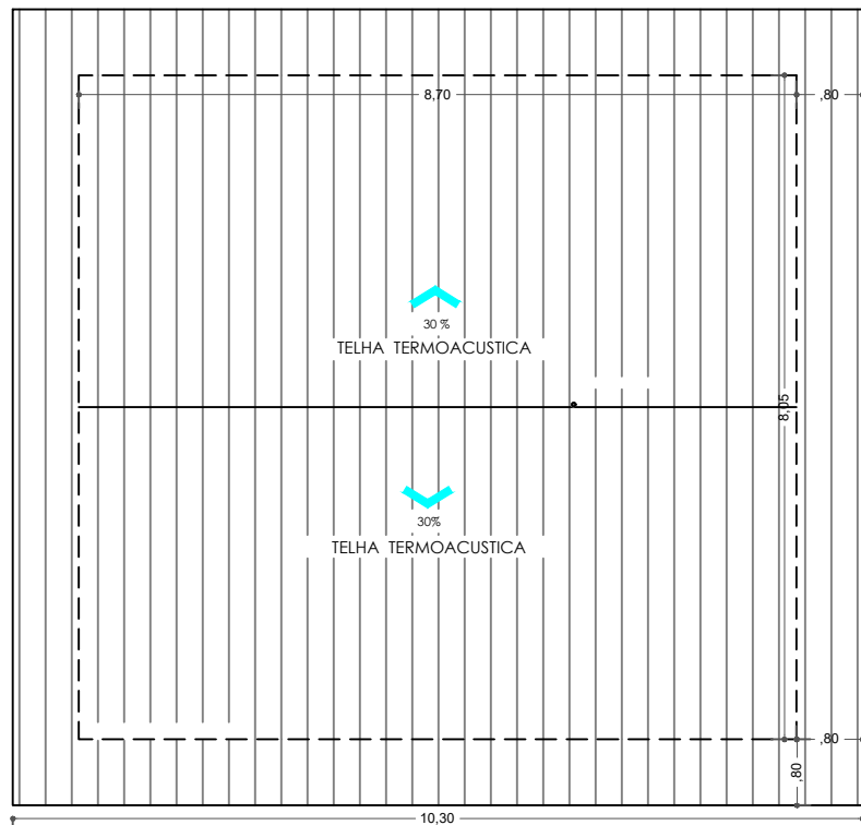
PLANTA DE COBERTURA
