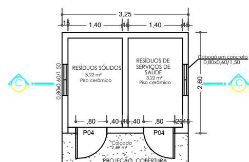
PLANTA BAIXA - ABRIGO DE RESÍDUOS
