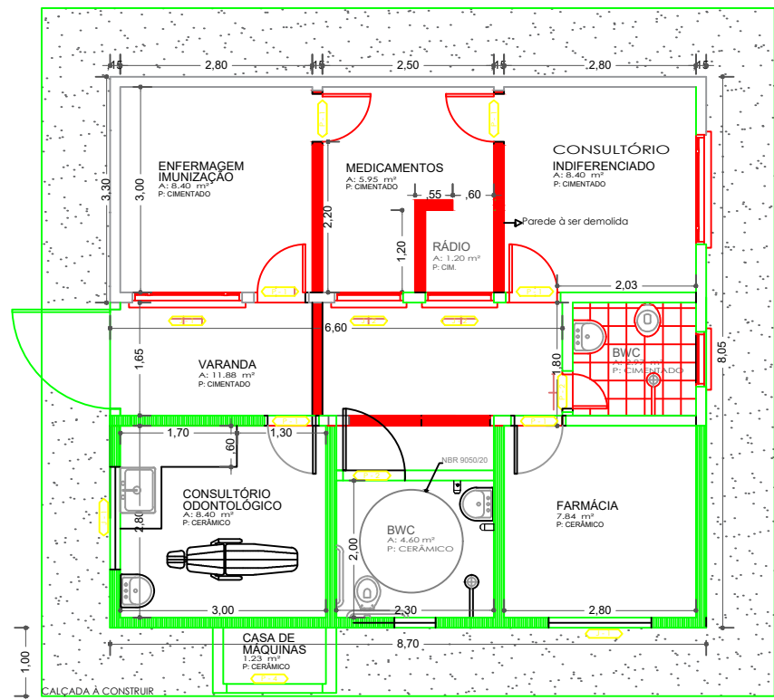
PLANTA BAIXA - CONSTRUIR / DEMOLIR
