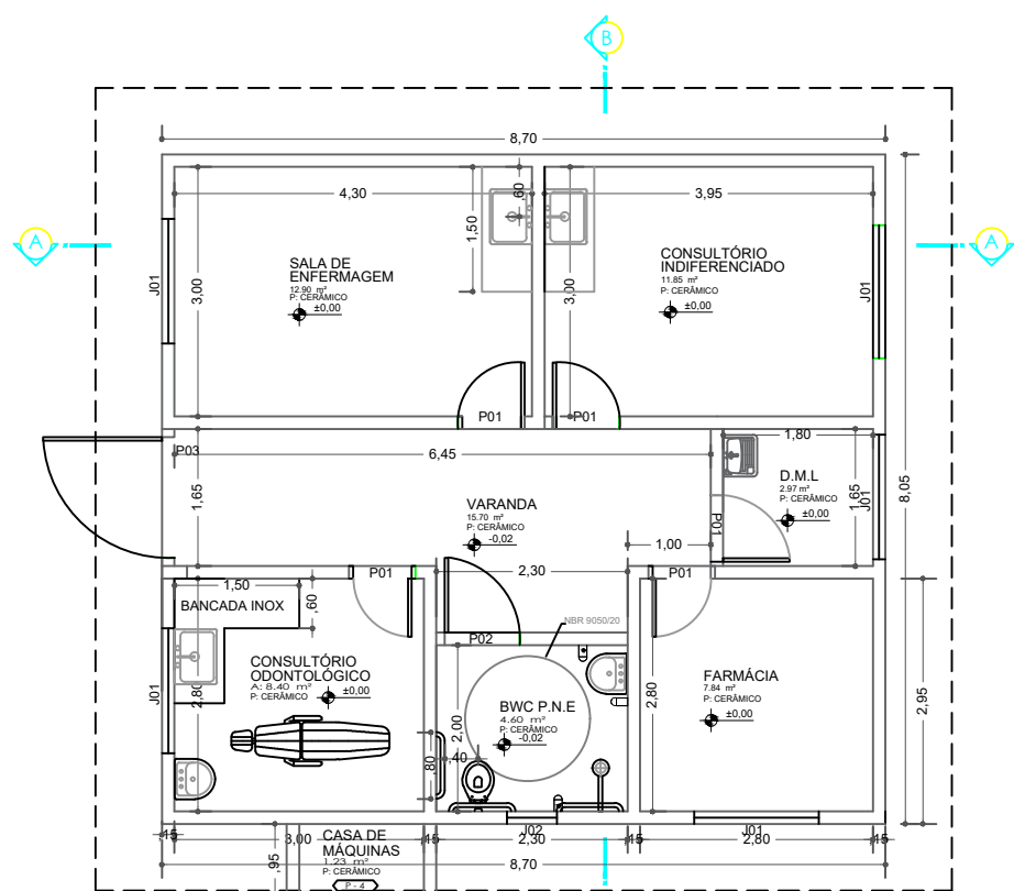
PLANTA BAIXA - AMPLIAÇÃO
