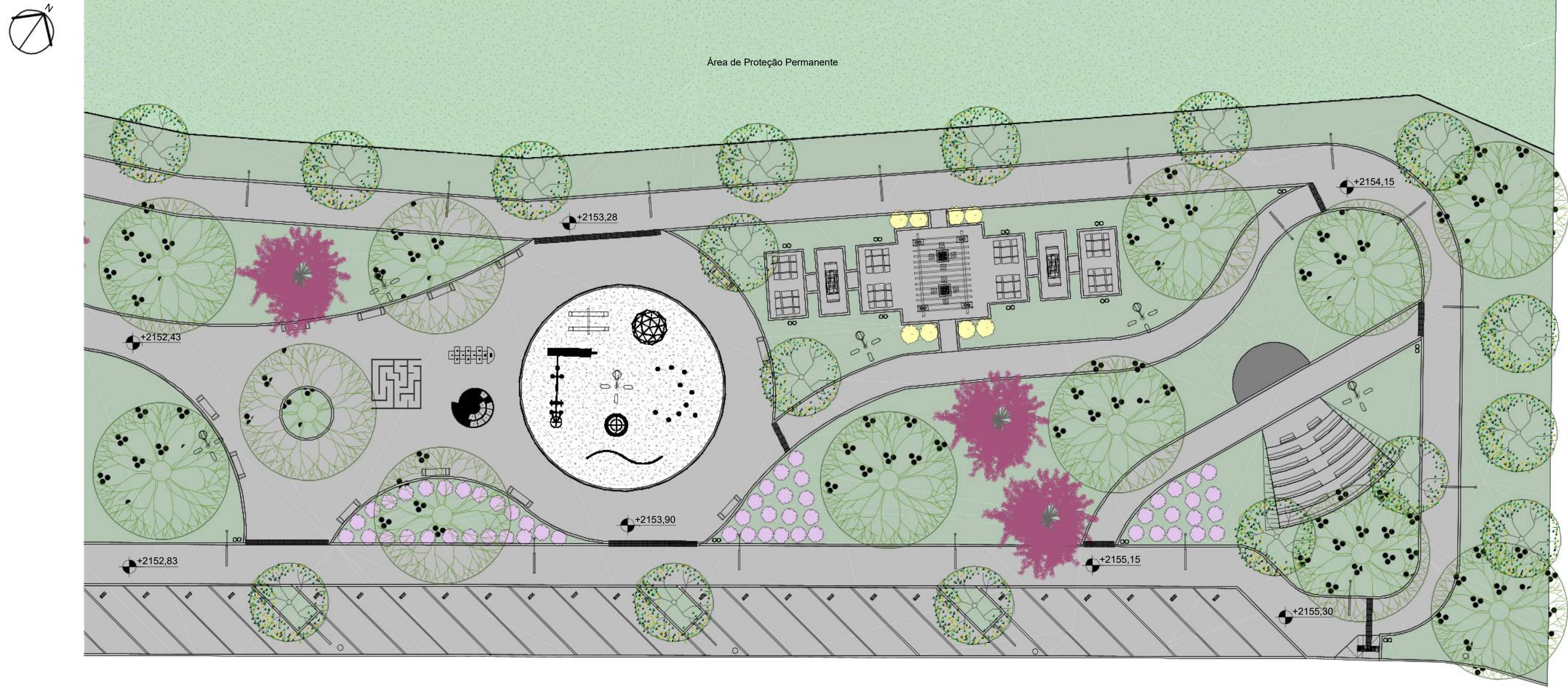
2 PAISAGISMO - TRECHO 03 ESCALA 1:250
