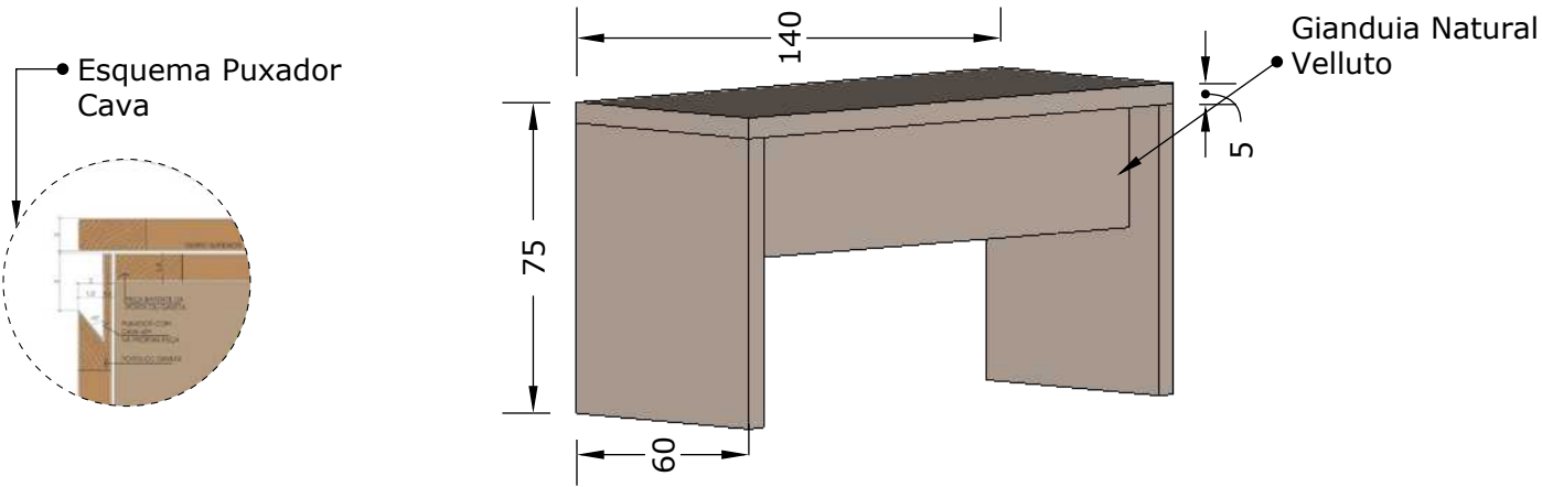
VISTA ISOMÉTRICA
