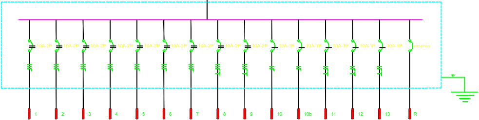
DIAGRAMA UNIFILAR - QDLF-08 (Guarita)
