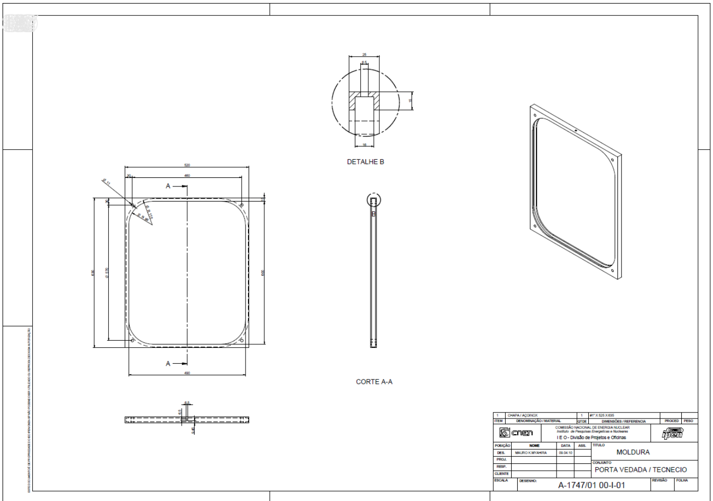
Figura 05 - Desenho A-1747/01 00-I-01.
