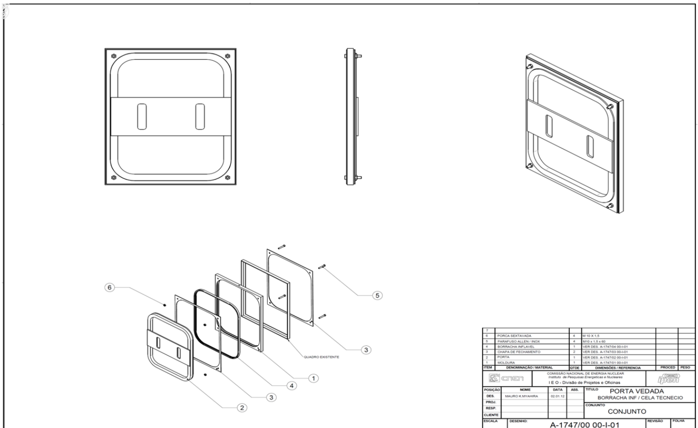
Figura 04 - Desenho A-1747/00 00-I-01
