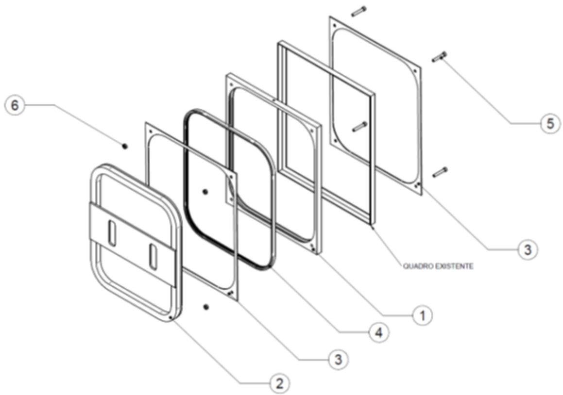
Figura 01 - Esboço do Equipamento e Componentes.
