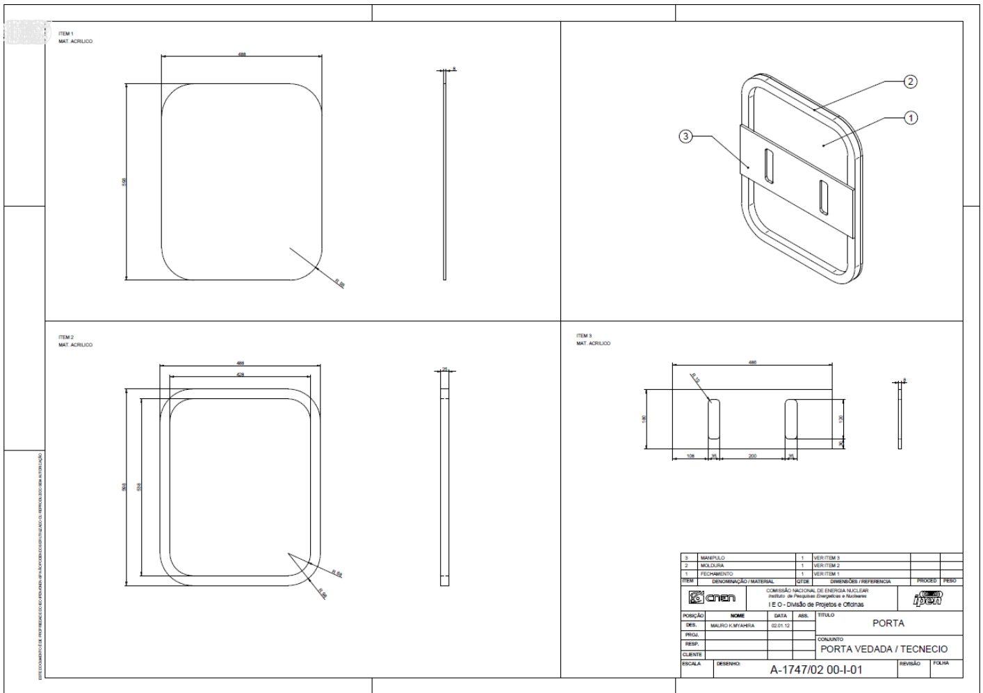
Figura 06 - Desenho A-1747/02 00-I-01.
