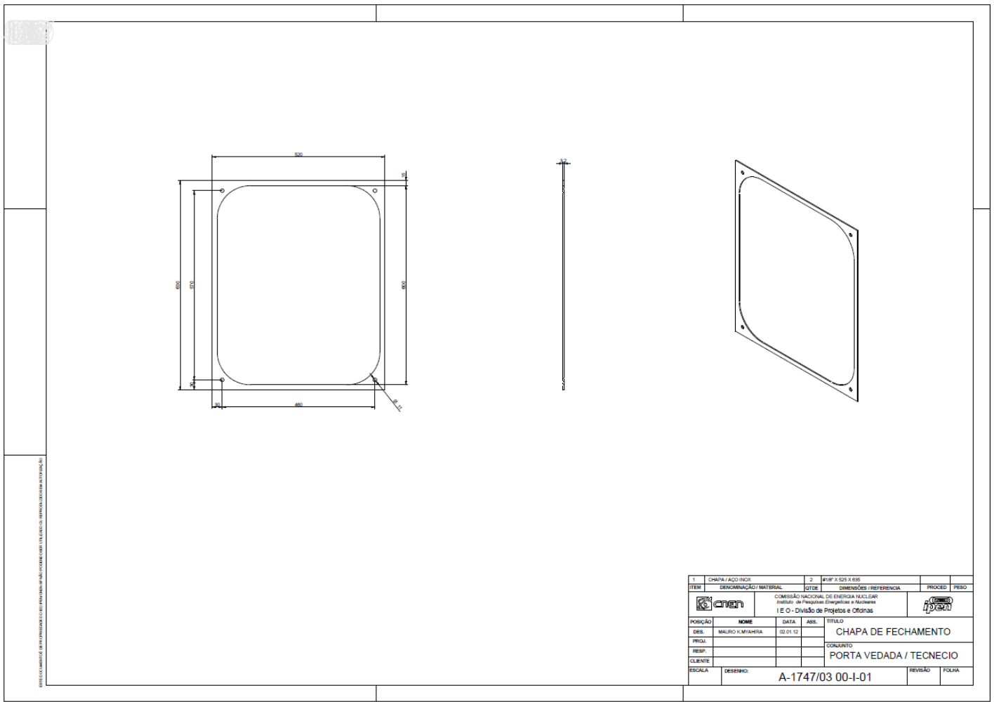
Figura 07 - Desenho A-1747/03 00-I-01.
