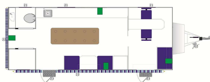
UNIDADE MÓVEL TRAILER FLAMINGO MÉDICO/ATENDIMENTO PLANTA BAIXA
