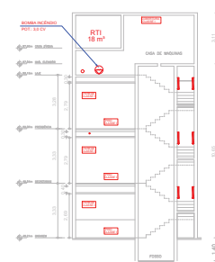
CORTE CC ESC: 1:100
