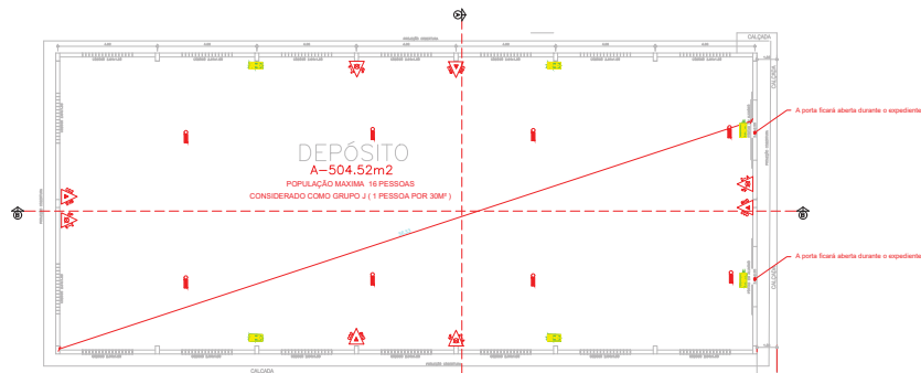
PLANTA BAIXA DEPÓSITO ESC: 1:100
