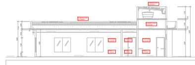
CORTE BB — ALOJAMENTO ESC: 1:100
