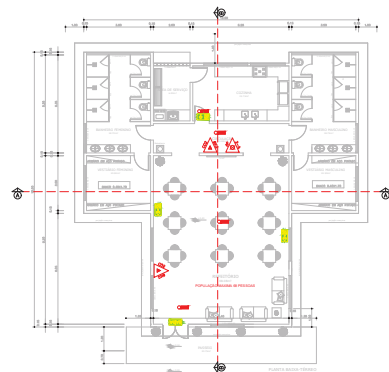
PLANTA BAIXA — ALOJAMENTO ESC: 1:100
