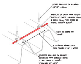
DET.040 SEM ESCALA
