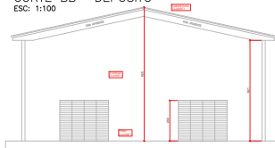
CORTE AA – DEPOSITO ESC: 1:100
