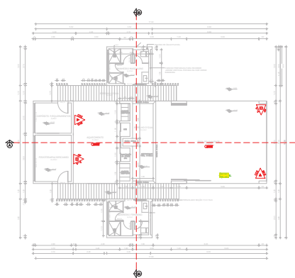
PLANTA BAIXA ESPAÇO DE CONVIVÊNCIA ESC: 1:100
