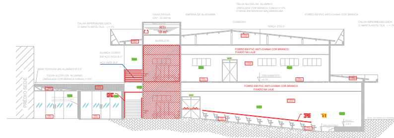
Corte CC - Predio Anexo
