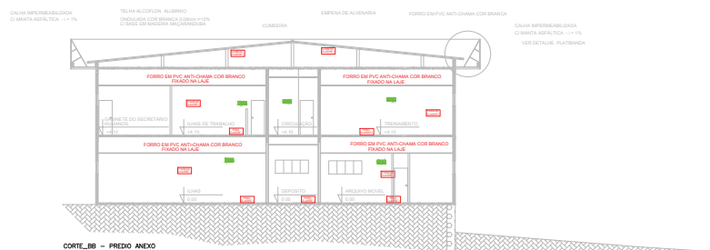
Corte BB - Predio Anexo
