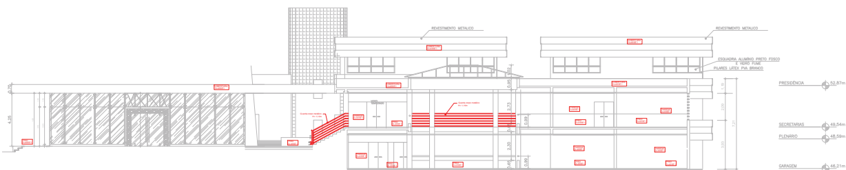
CORTE AA - SEDE ESC: 1:100
