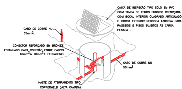
DET.010 SEM ESCALA
