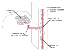
DET.03A SEM ESCALA
