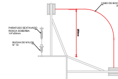
DET.02A SEM ESCALA
