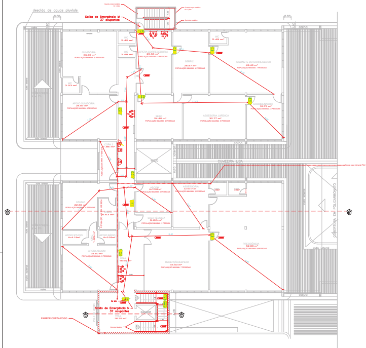
PLANTA BAIXA 2º PAVIMENTO ESC: 1:100
