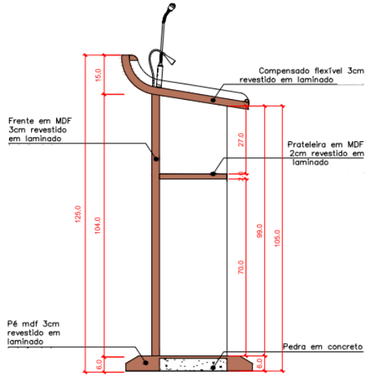
CORTE AA Escala 1/10
