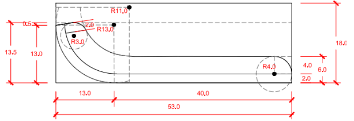
MARCAÇÃO CURVATURAS 02 Escala 1/5
