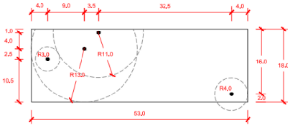
MARCAÇÃO CURVATURAS 01
