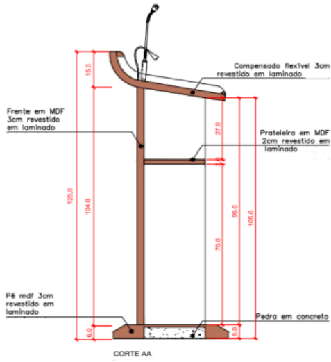
CORTE AA
