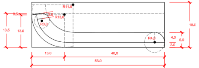
MARCAÇÃO CURVATURAS 02
