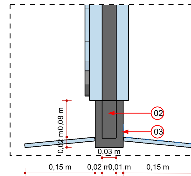
02 DET. DO SISTEMA DA BASE ESC.: 1/15
