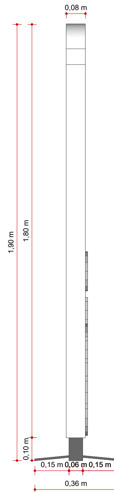
04 VISTA LATERAL ESC.:.....1/30
