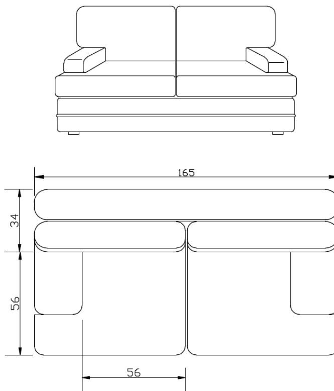
VISTA SUPERIOR
