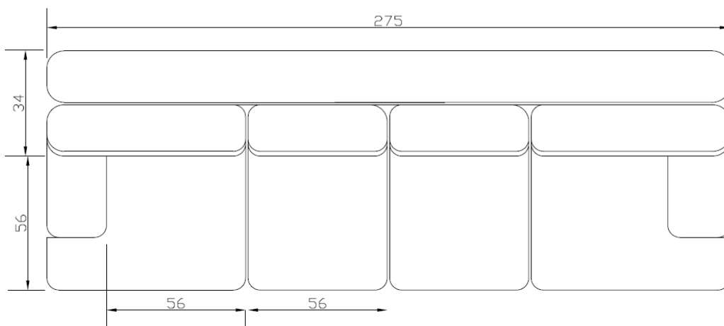
VISTA SUPERIOR
