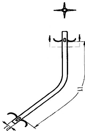
Fig.4 Cateter de drenagem biliar com quatro abas laterais
