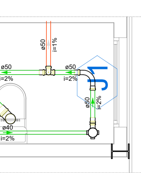
DETALHE SAN-2 1:25
