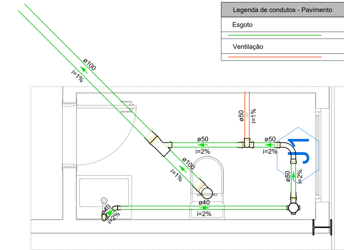
DETALHE SAN-1 1:25
