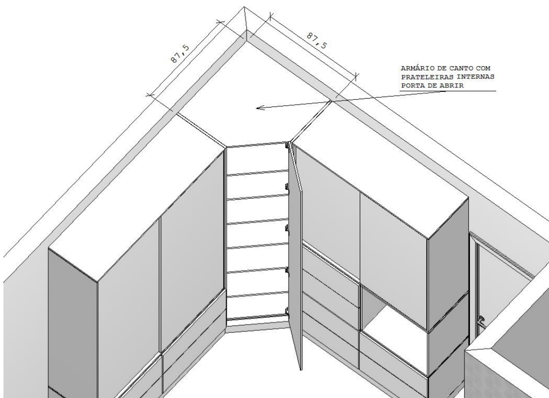
PORTA DE ABRIR NO ARMÁRIO DO CANTO COM PRATELEIRAS INTERNAS (CAIXA MDF 18MM, FRENTE MDF 15MM)
