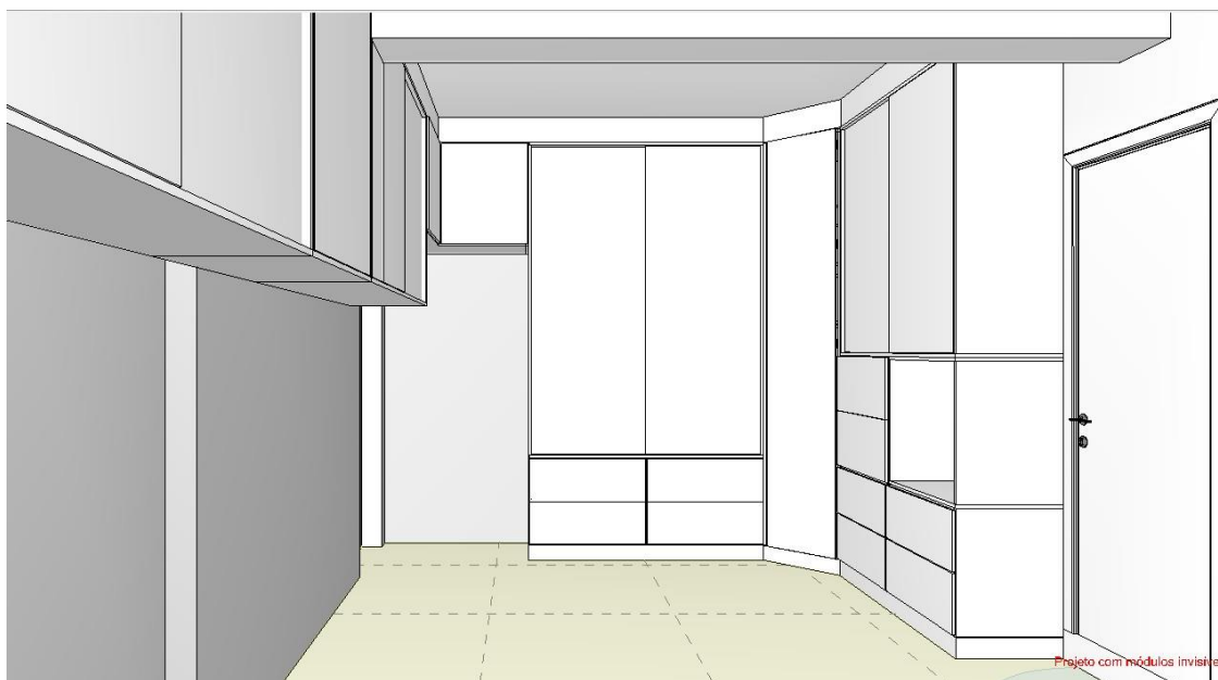
ARMÁRIO GRANDE COM GAVETEIROS COM CORREDIÇAS TELESCÓPICAS, PORTAS DE CORRER NA PARTE SUPERIOR. CAIXAS E PORTAS DE CORRER EM MDF DE 18MM, FRENTES DE GAVETAS EM MDF 15MM
