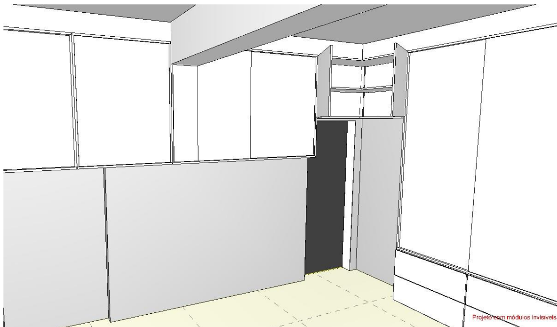
PORTA DE ABRIR NO ARMÁRIO DO CANTO COM PRATELEIRA INTERNA (CAIXA MDF 18MM, FRENTE MDF 15MM)
