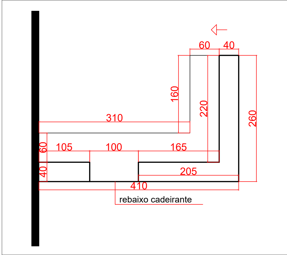
PLANTA BAIXA BALÇÃO RECEPÇÃO ENTRADA
