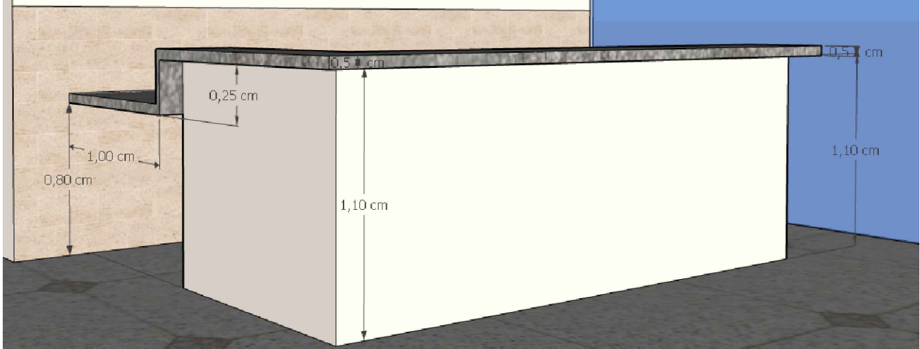
ELEVAÇÕES FRONTAIS/LATERAIS
