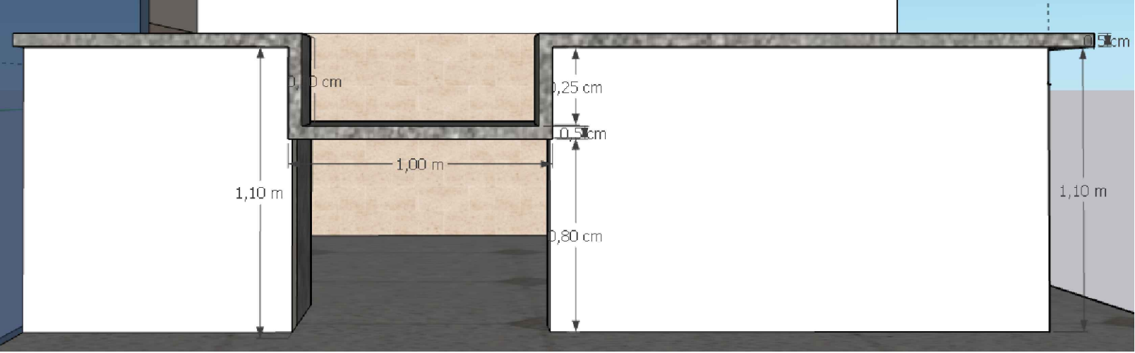
ELEVAÇÕES FRONTAIS/LATERAIS
