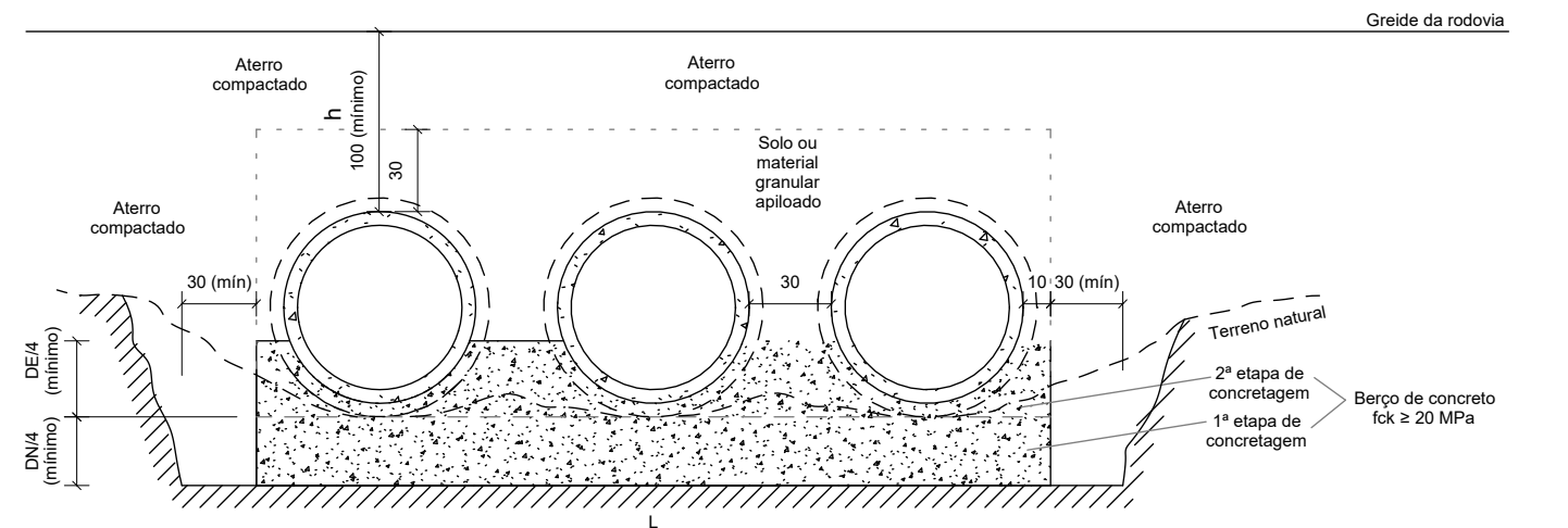
Seção transversal - Linha tripla Sem escala
