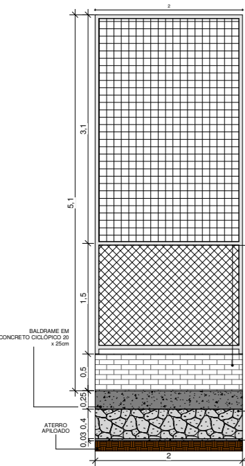
DET. MURETA E ALAMBRADO 02 ESC. 1:25
