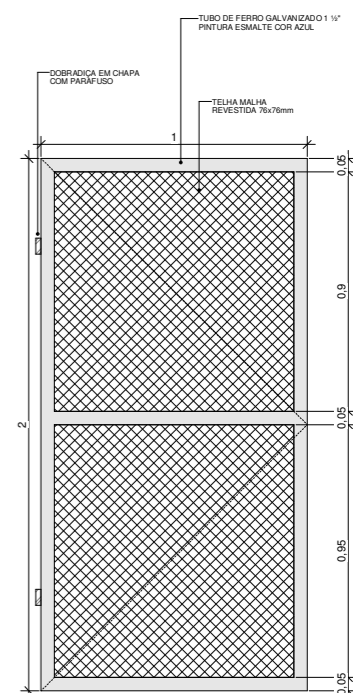
DET. PORTA ENTRADA ESC. 1:10
