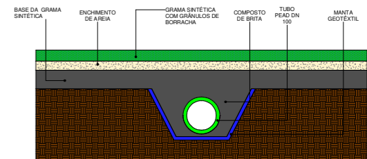
DET. DRENAGEM ESC. 1:10
