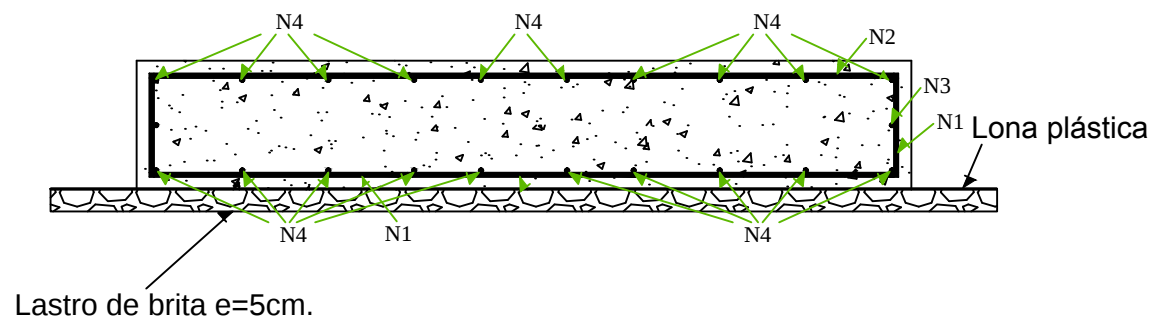
1 CORTE B-B S/ESCALA
