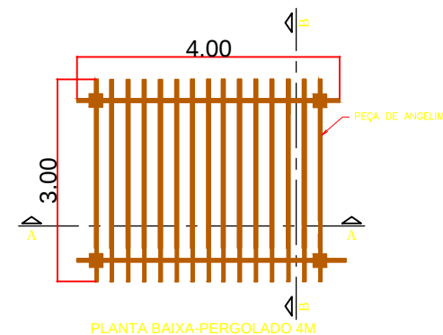
DET. PERGOLADO ESC. S/ESCALA
