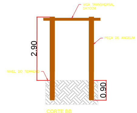
CORTE BB
