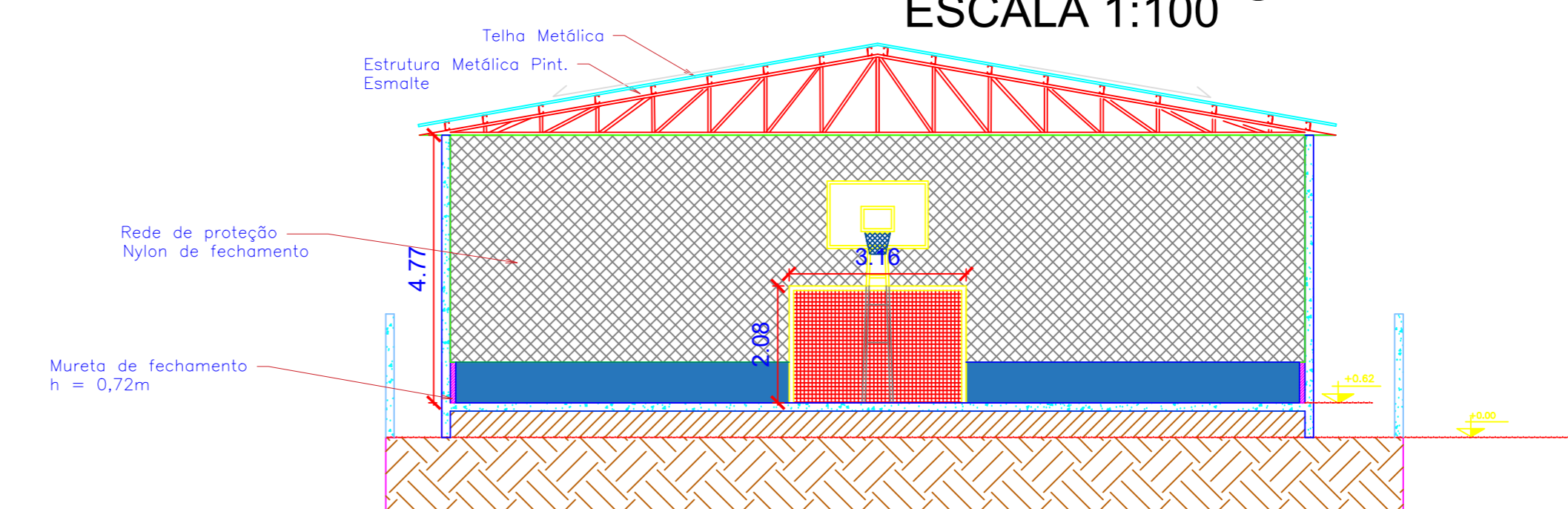
COTE AA ESCALA 1:100
