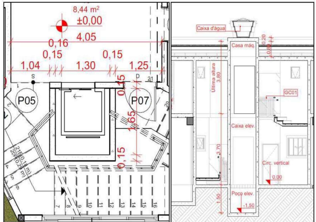
Figura 01 – Recorte da planta baixa e corte da caixa de subida do elevador, respectivamente.
