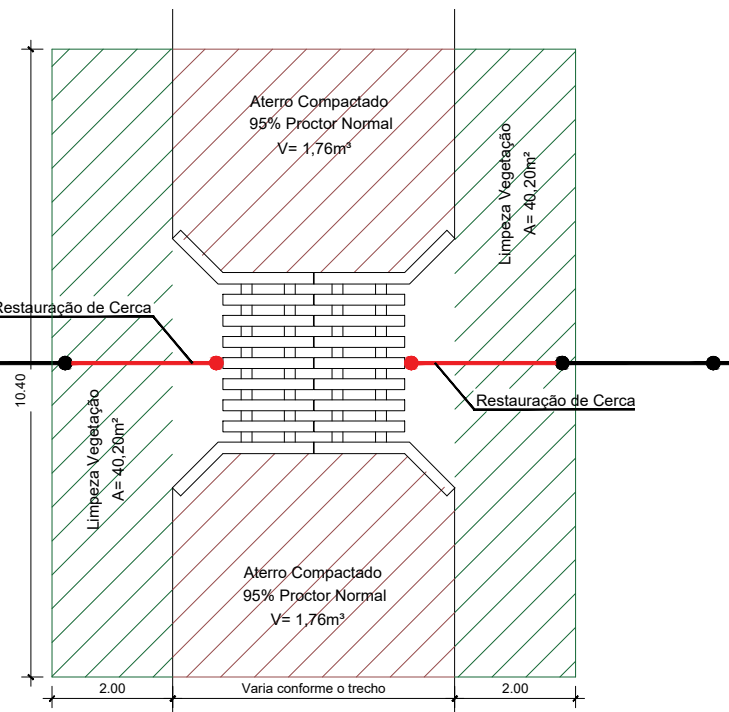
PLANTA DE LOCAÇÃO ESCALA: 1/25
