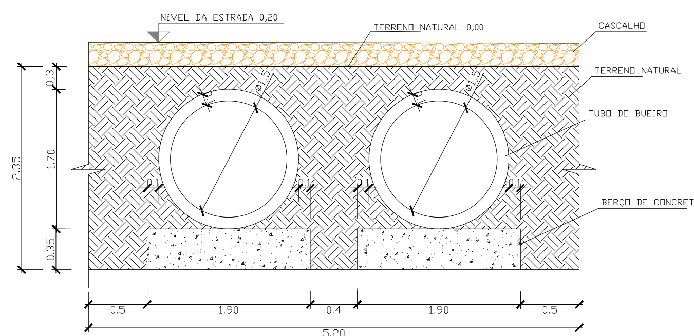
CROQUI DO BUEIRO NO TERRENO
