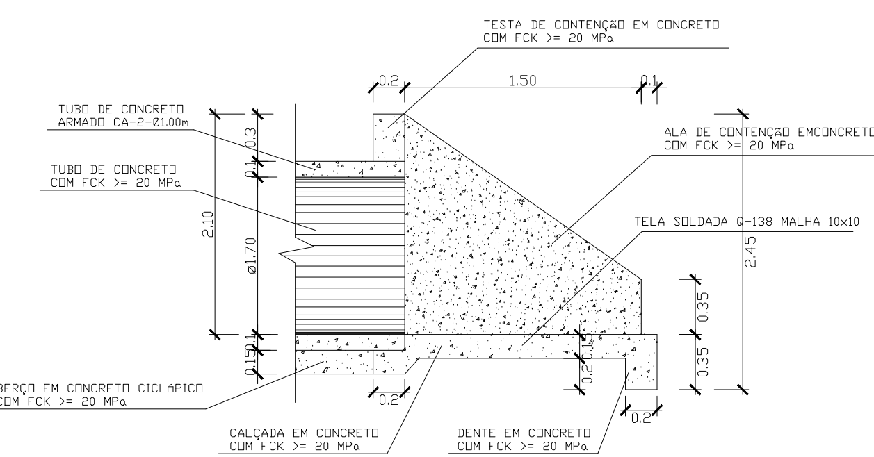
VISTA LATERAL BICA DE BUEIRO DUPLO DE CONCRETO DE Ø1.00m S/ESCALA
