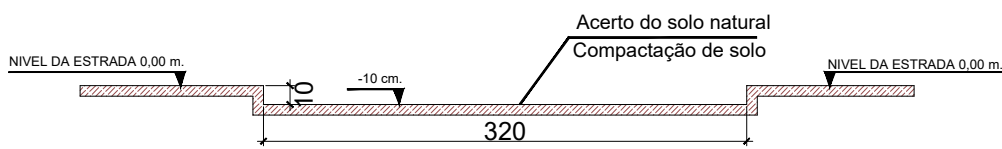
CORTE ESCAVAÇÃO ESCALA: 1/25
