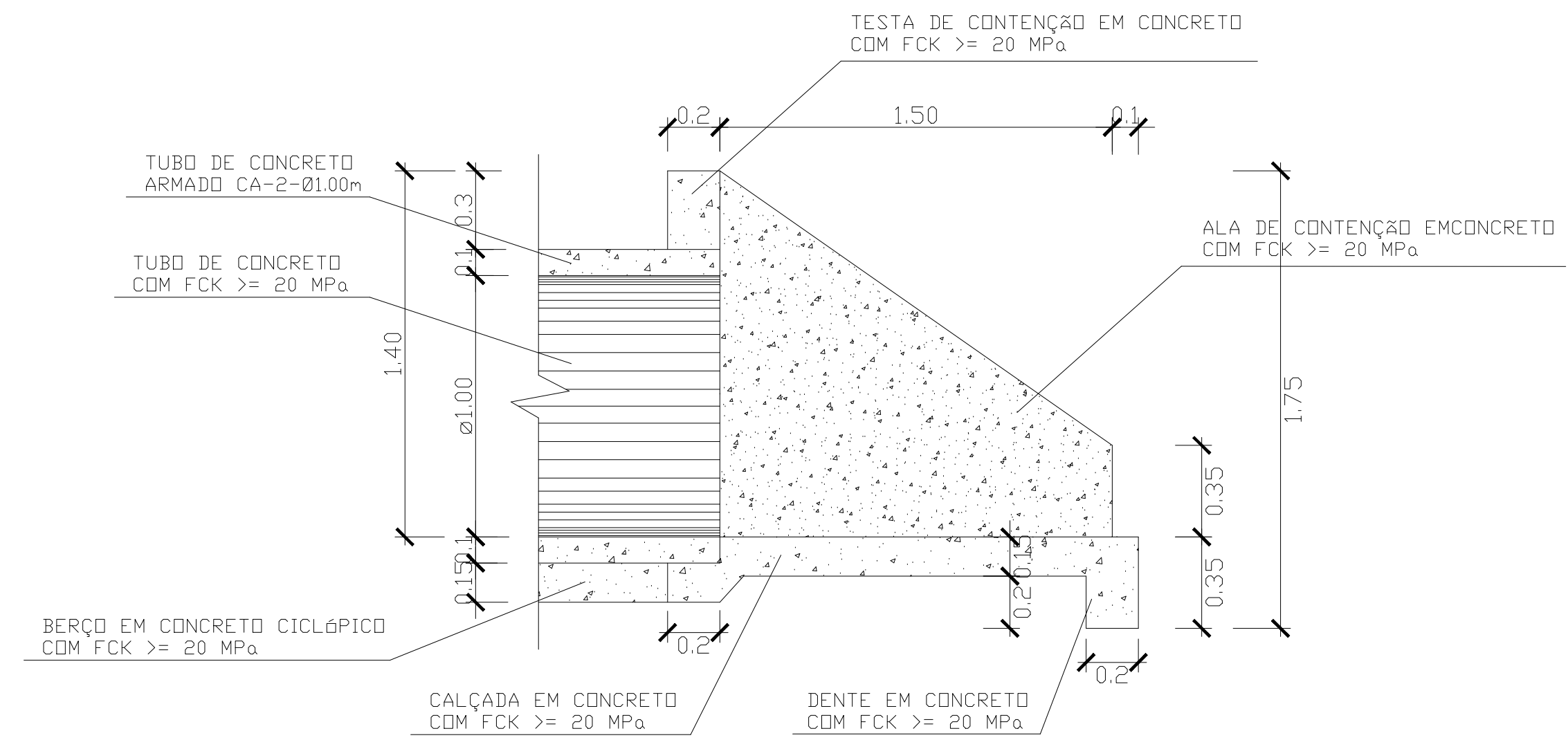
VISTA LATERAL
