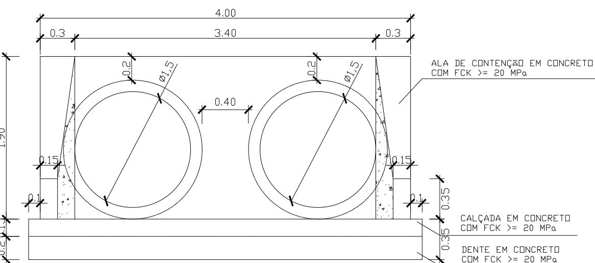
VISTA FRONTAL - ENTRADA
