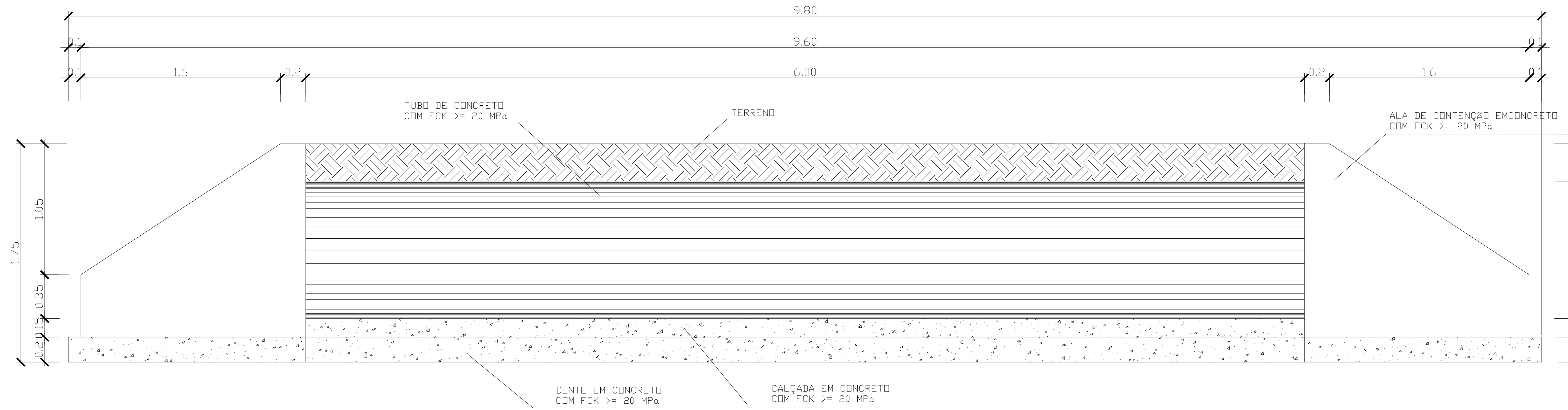
DETALHAMENTO DO BUEIRO - LONGITUDINAL
