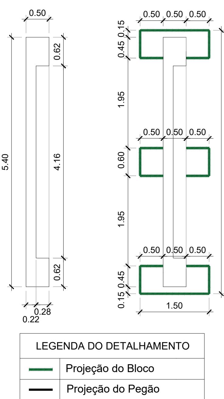
Pegão 1 e 2 h = 2,79 m
