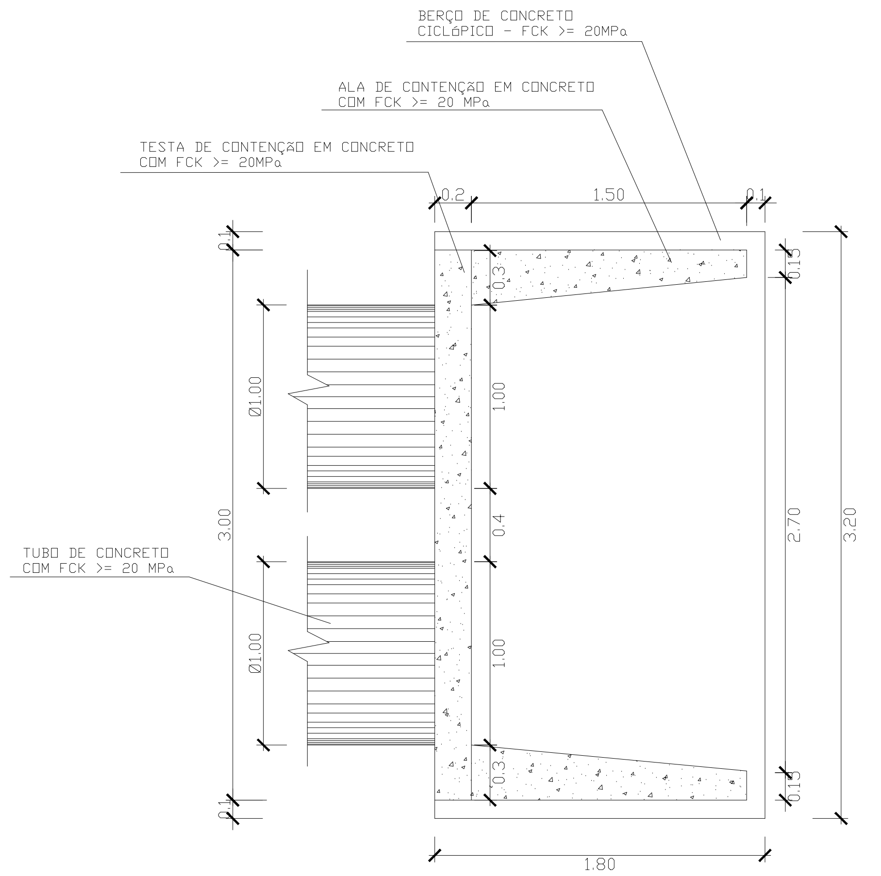
PLANTA BAIXA
