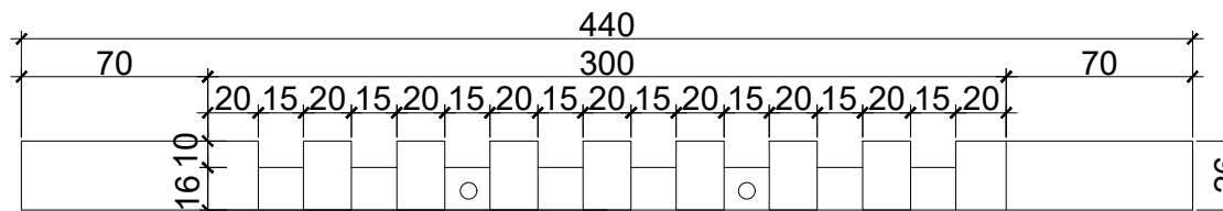
CORTE ESCALA: 1/25
