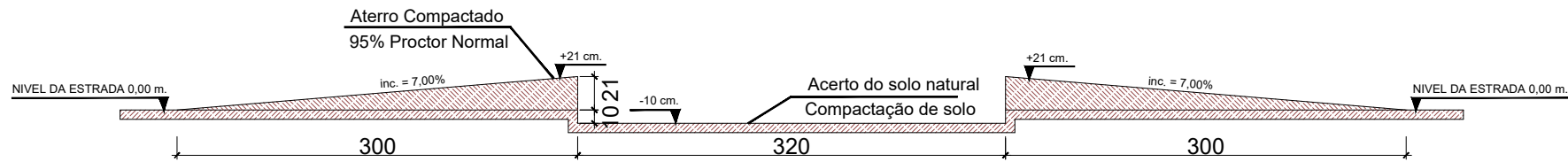
CORTE ATERRO ESCALA: 1/25
