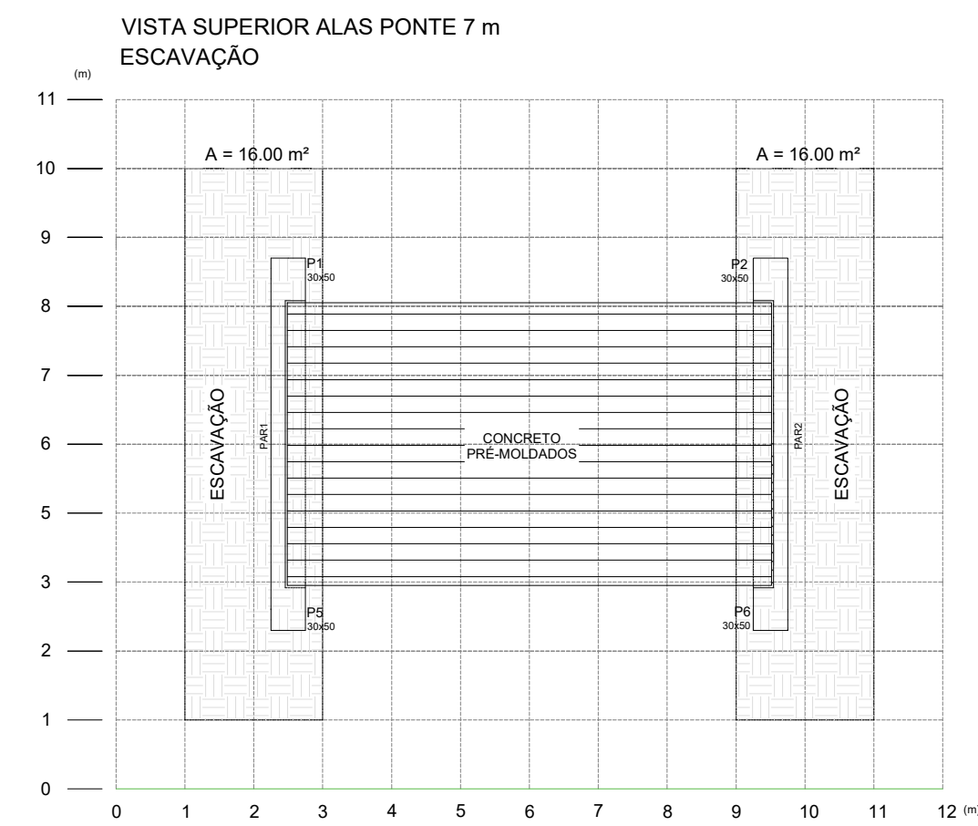
ESCAVAÇÃO E ATERRO ESC: 1/50
