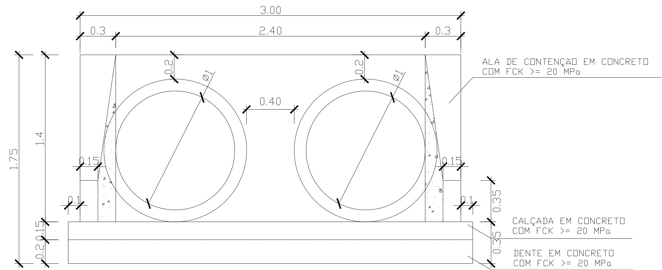
VISTA FRONTAL - ENTRADA
