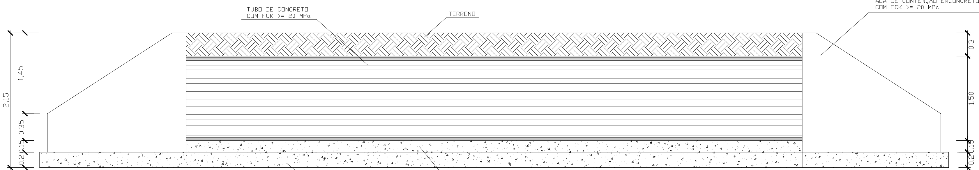
CORTE DO BUEIRO - LONGITUDINAL
