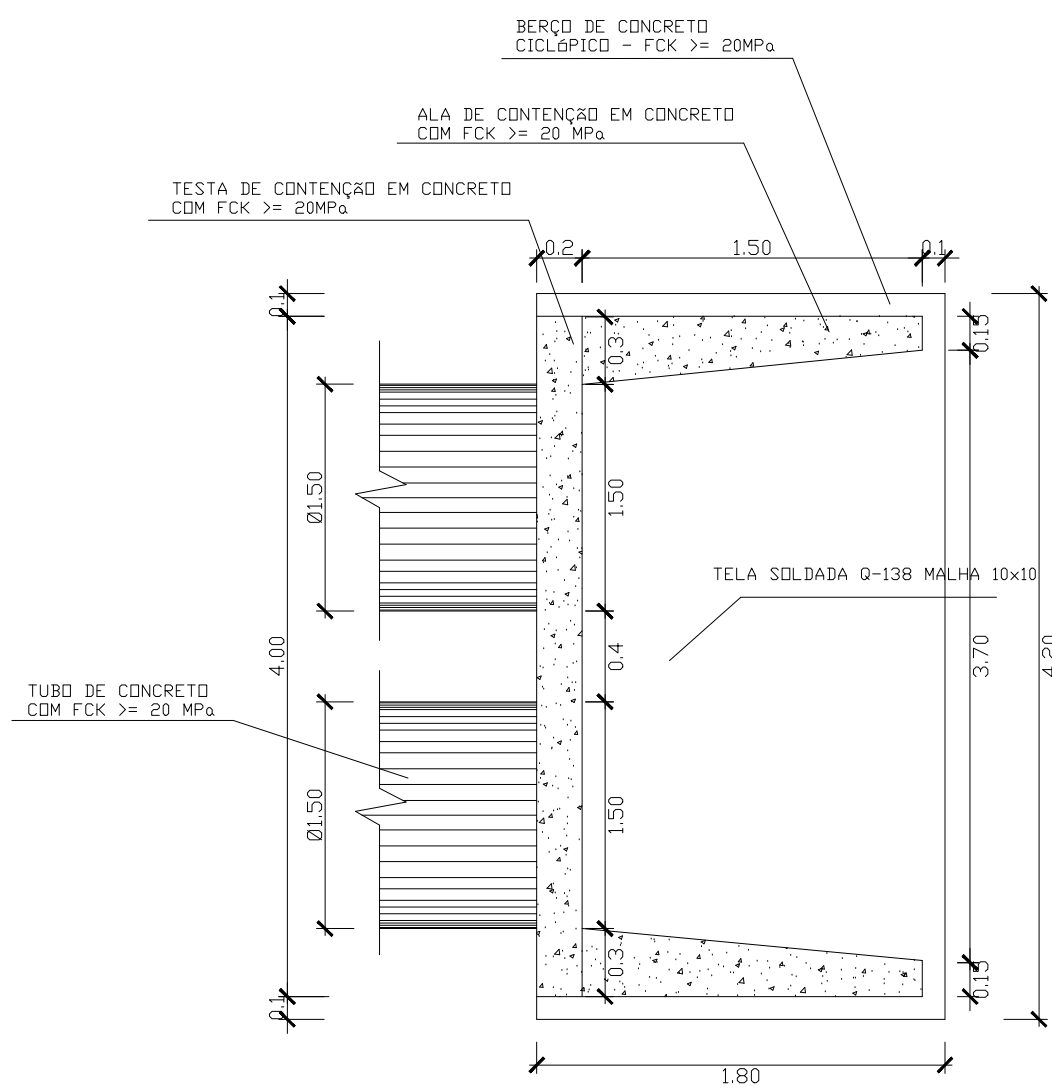
PLANTA BAIXA BICA DE BUEIRO DUPLO DE CONCRETO DE Ø1.00m S/ESCALA
