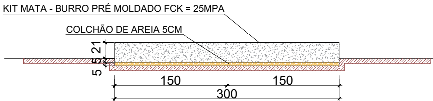
DETALHAMENTO ESCALA: 1/25
