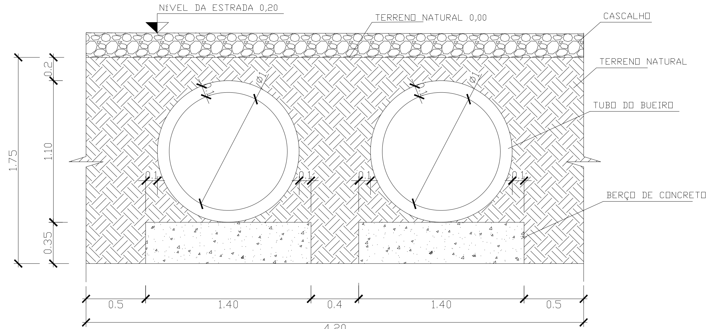
CROQUI DO BUEIRO NO TERRENO
