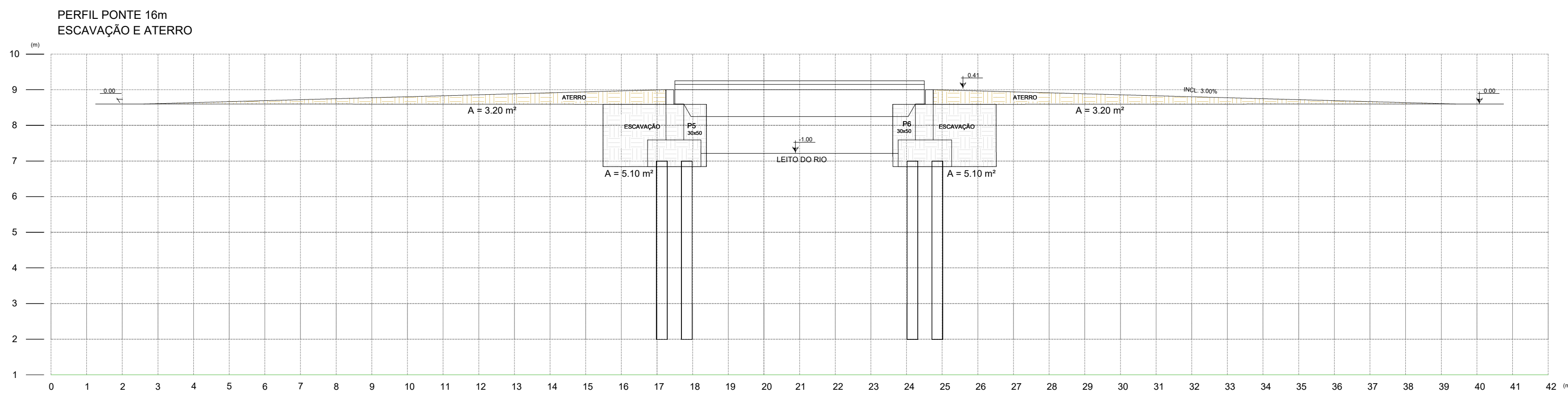
NOTA DE SERVIÇO DE ATERRO E ESCAVAÇÃO TOTAL - PONTE DE 16 M
