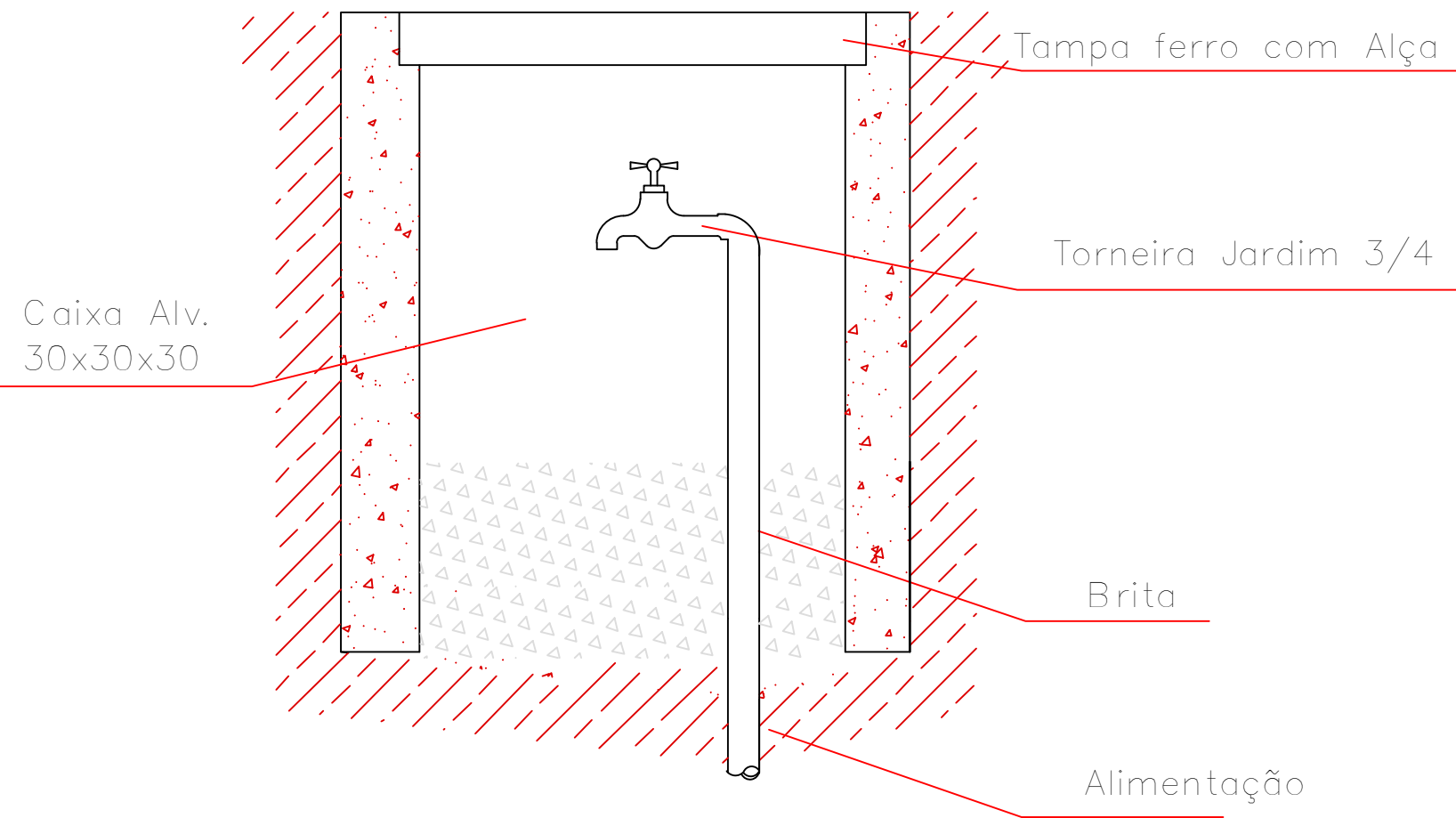
Detalhe da caixa de passagem em alvenaria (CX 10)
