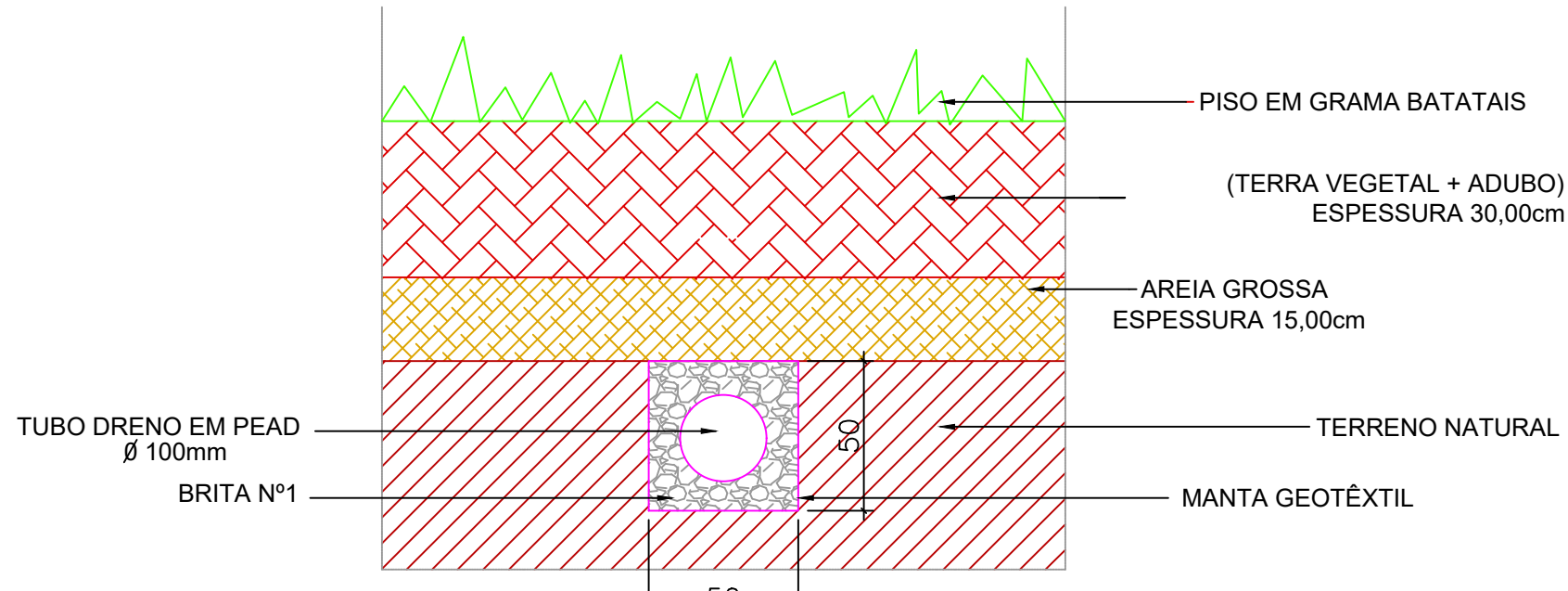
CORTE ESQUEMÁTICO EM GRAMA
