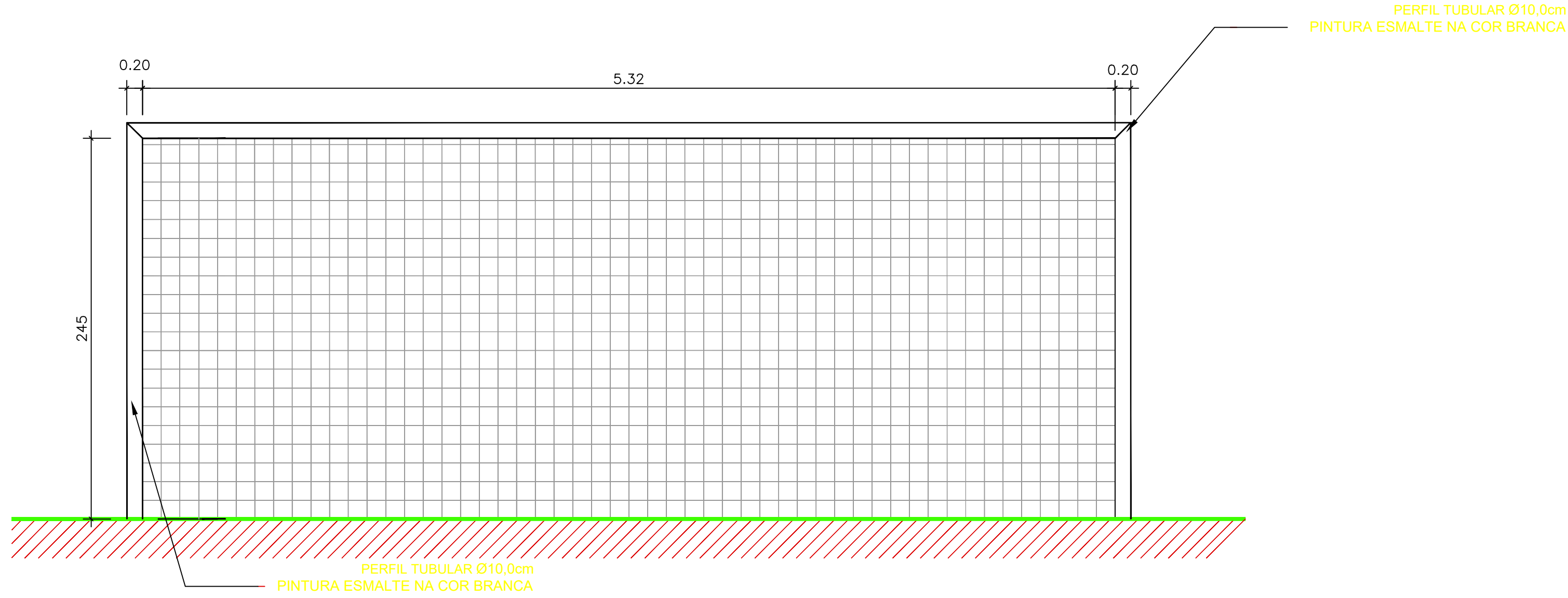
ELEVÇÃO DAS TRAVES DO GOL ESC 1/50
