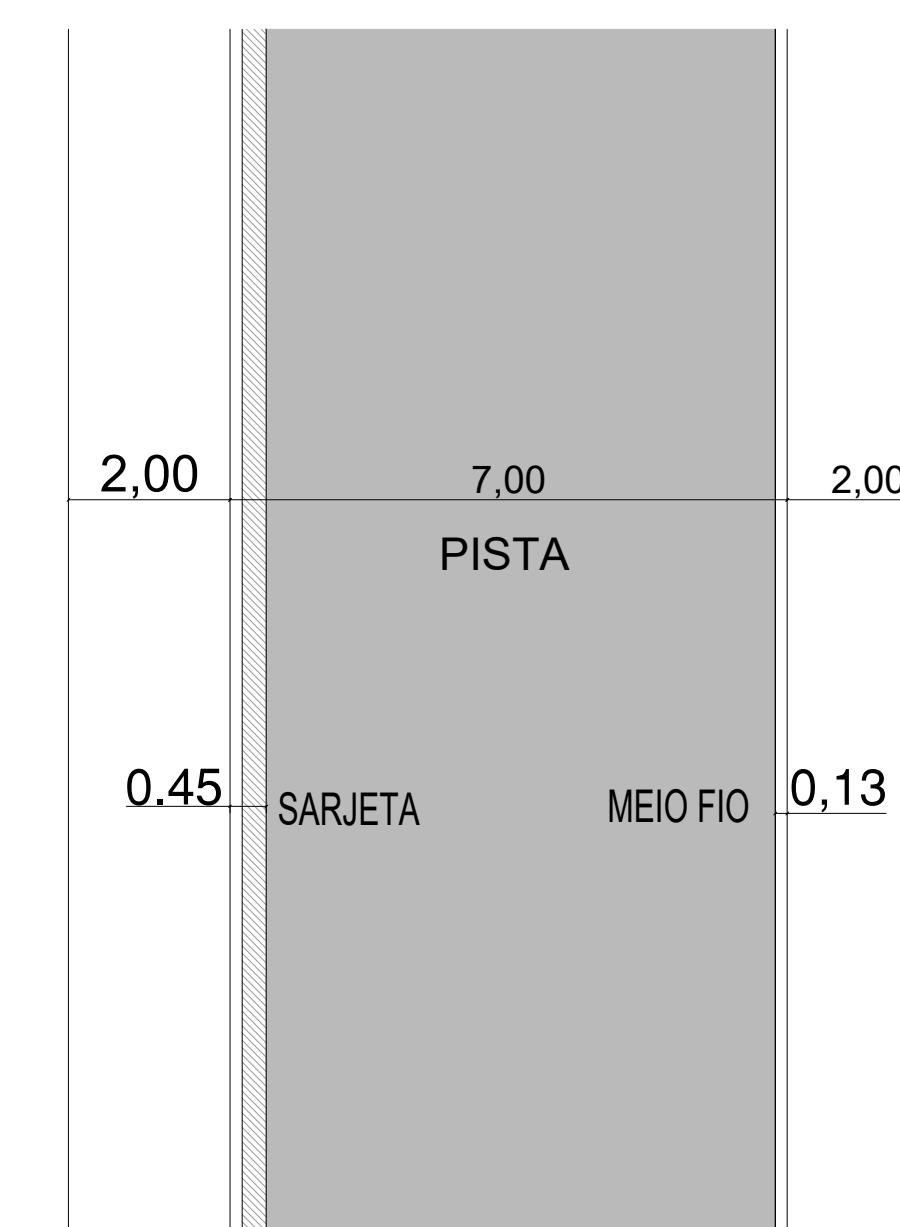
DETALHE SUPERIOR BASEADO NAS RUAS PAVIMENTADAS
