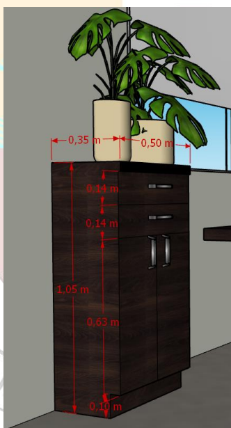
ARMÁRIO 07
