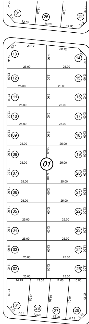
1 Planta de situação - Creche Escala: Sem escala
